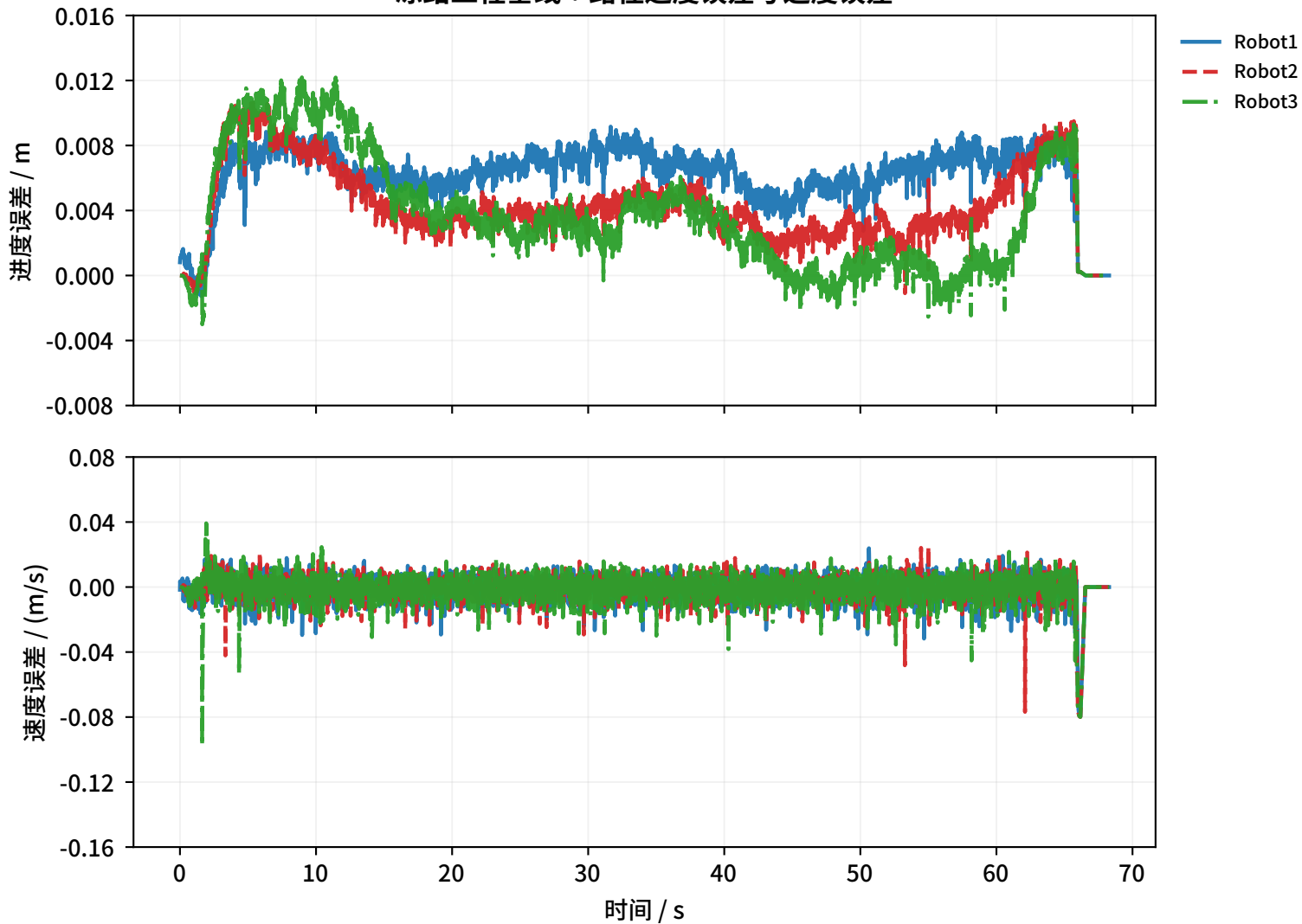
冻结工程基线：路径进度误差与速度误差
