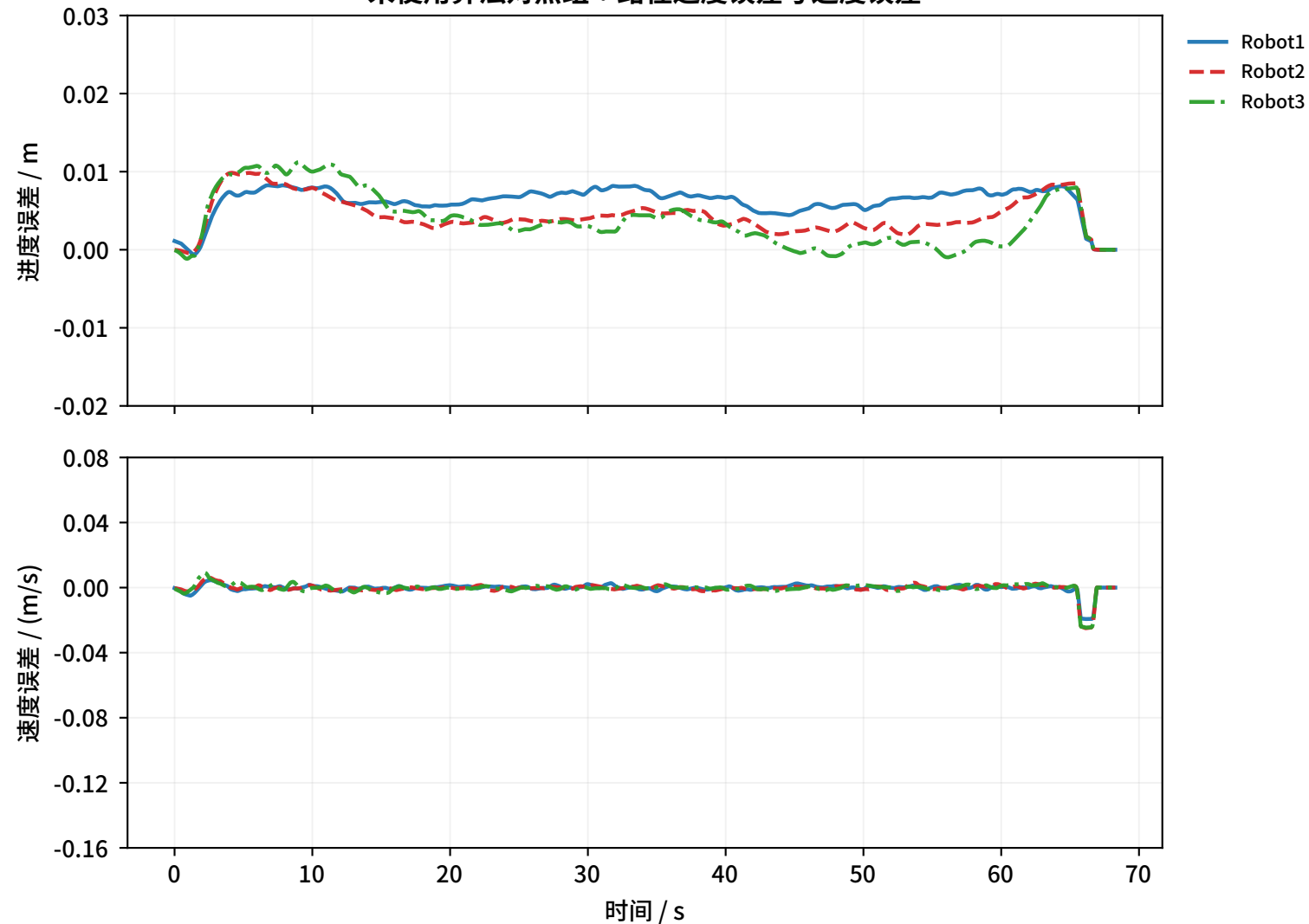
未使用算法对照组：路径进度误差与速度误差
