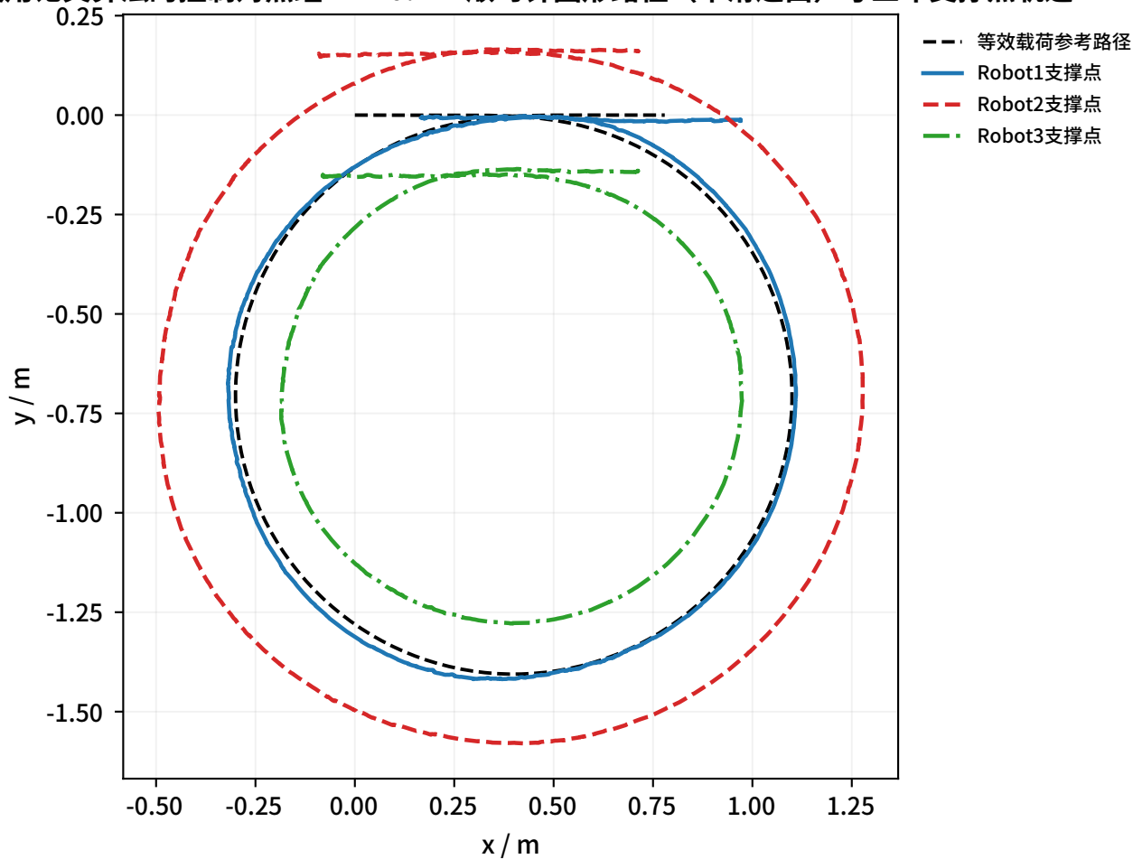
未使用论文算法的控制对照组：R=0.7 m顺时针圆形路径（平滑进出）与三车支撑点轨迹
