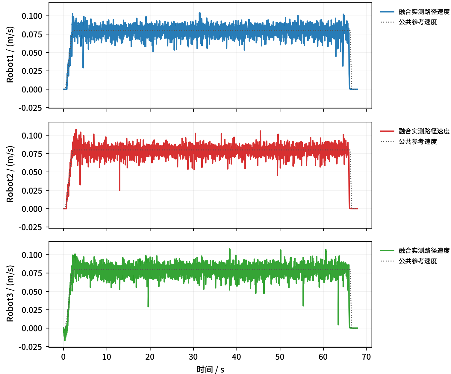
未使用论文算法的控制对照组：公共路径参考与实测路径速度（无M1动态边界）
