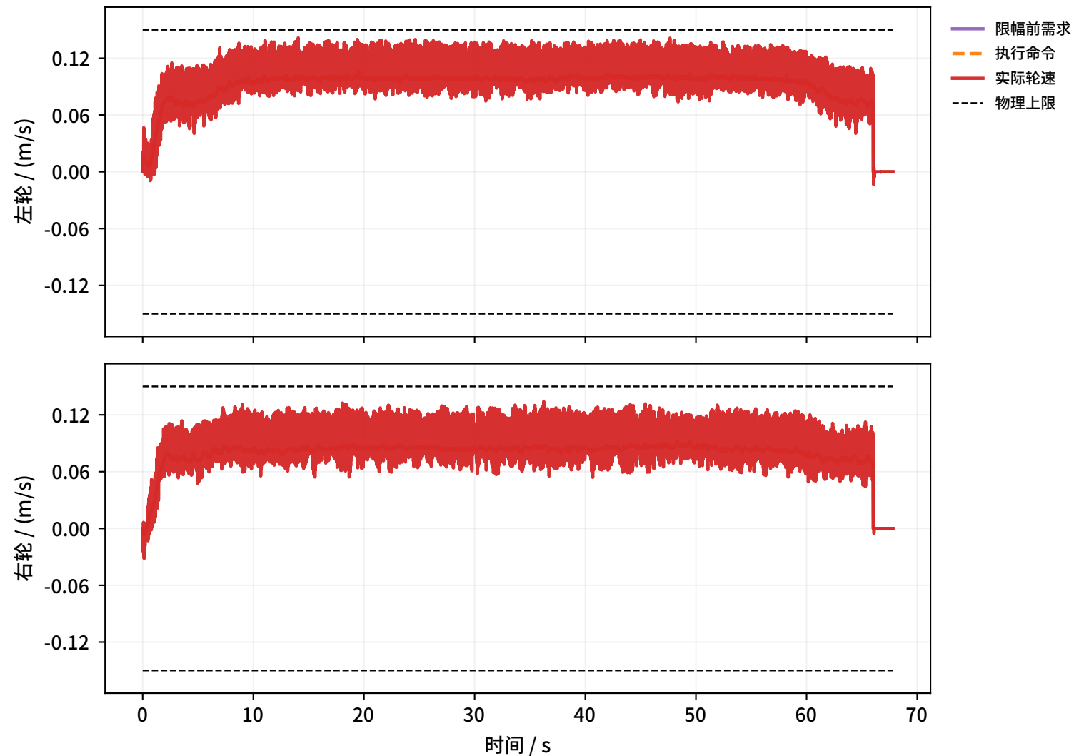
未使用论文算法的控制对照组：Robot2轮速需求、执行与反馈
