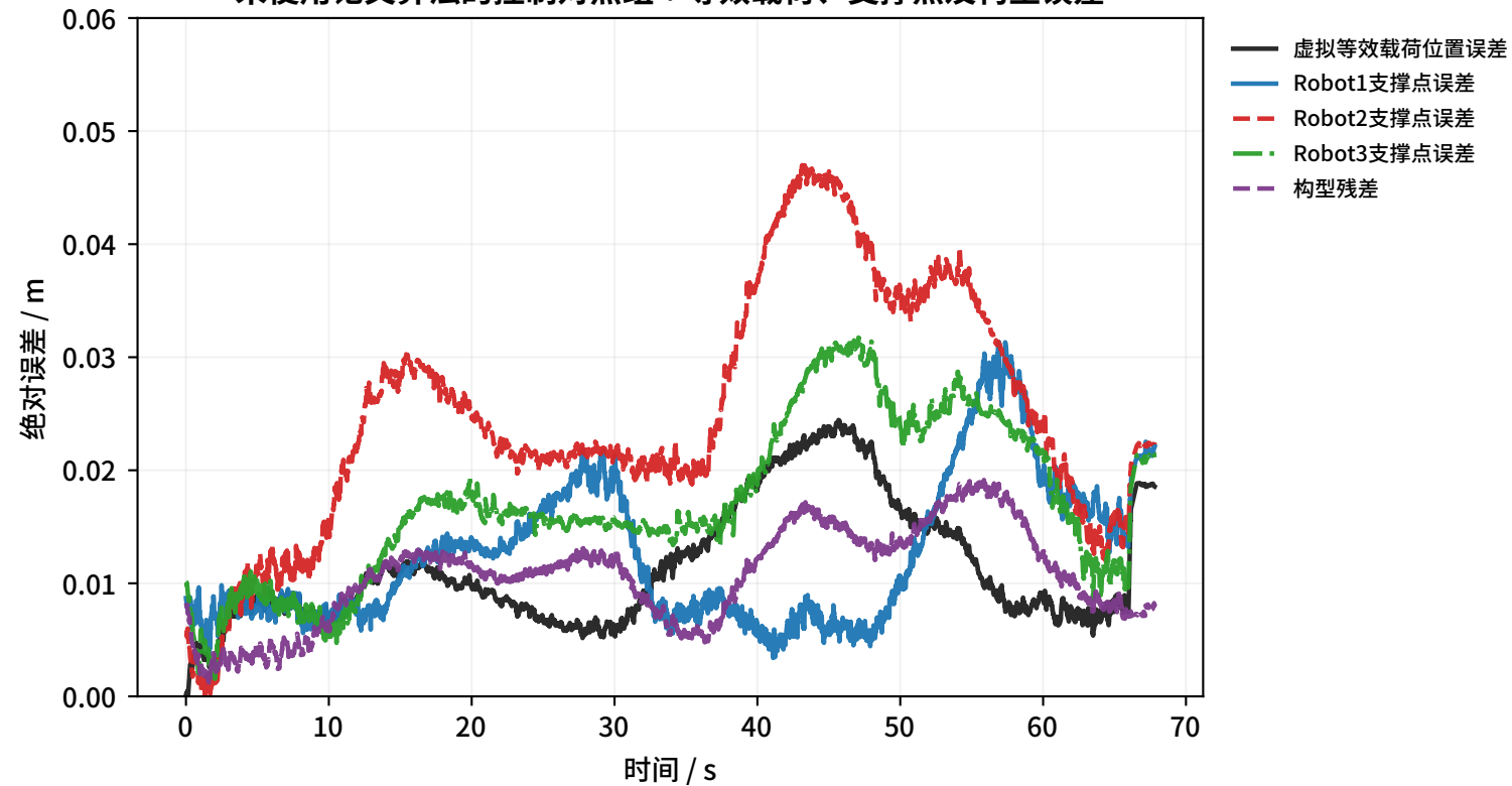
未使用论文算法的控制对照组：等效载荷、支撑点及构型误差
