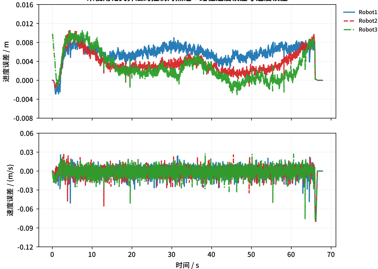
未使用论文算法的控制对照组：路径进度误差与速度误差
