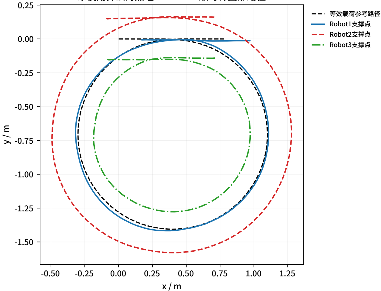
未使用算法对照组：R=0.7m顺时针圆形路径
