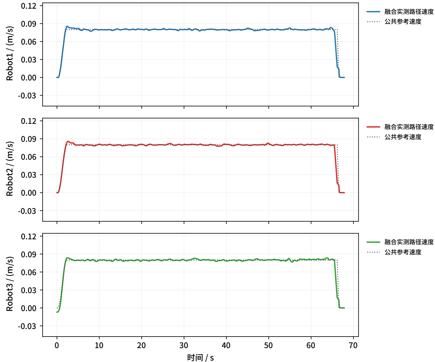
未使用算法对照组：公共路径参考与实测路径速度（无M1动态边界）
