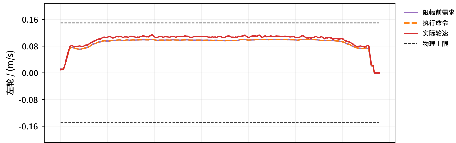
未使用算法对照组：Robot2轮速需求、执行与反馈
