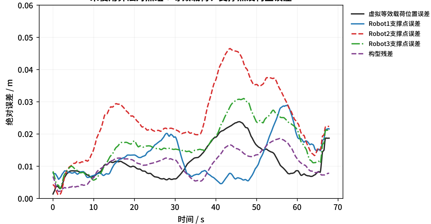
未使用算法对照组：等效载荷、支撑点及构型误差
