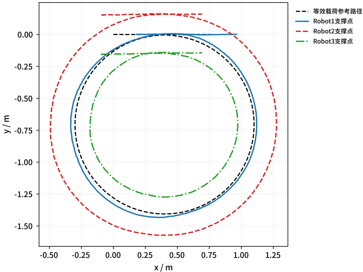
本文算法组 (Robot2降额) : R=0.7\text{m} 顺时针圆形路径
