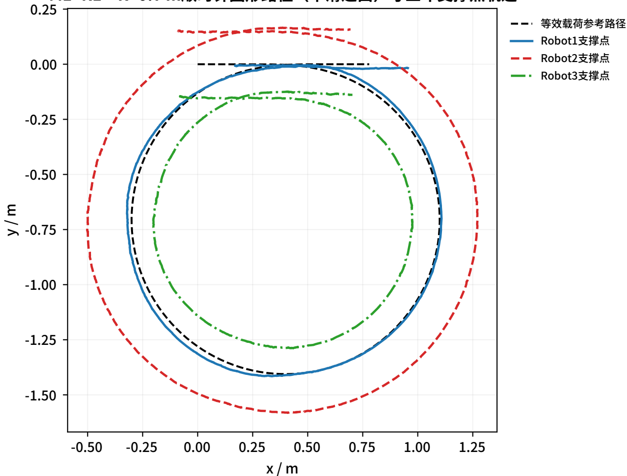
M1+R1 : R=0.7 m 顺时针圆形路径 (平滑进出) 与三车支撑点轨迹
