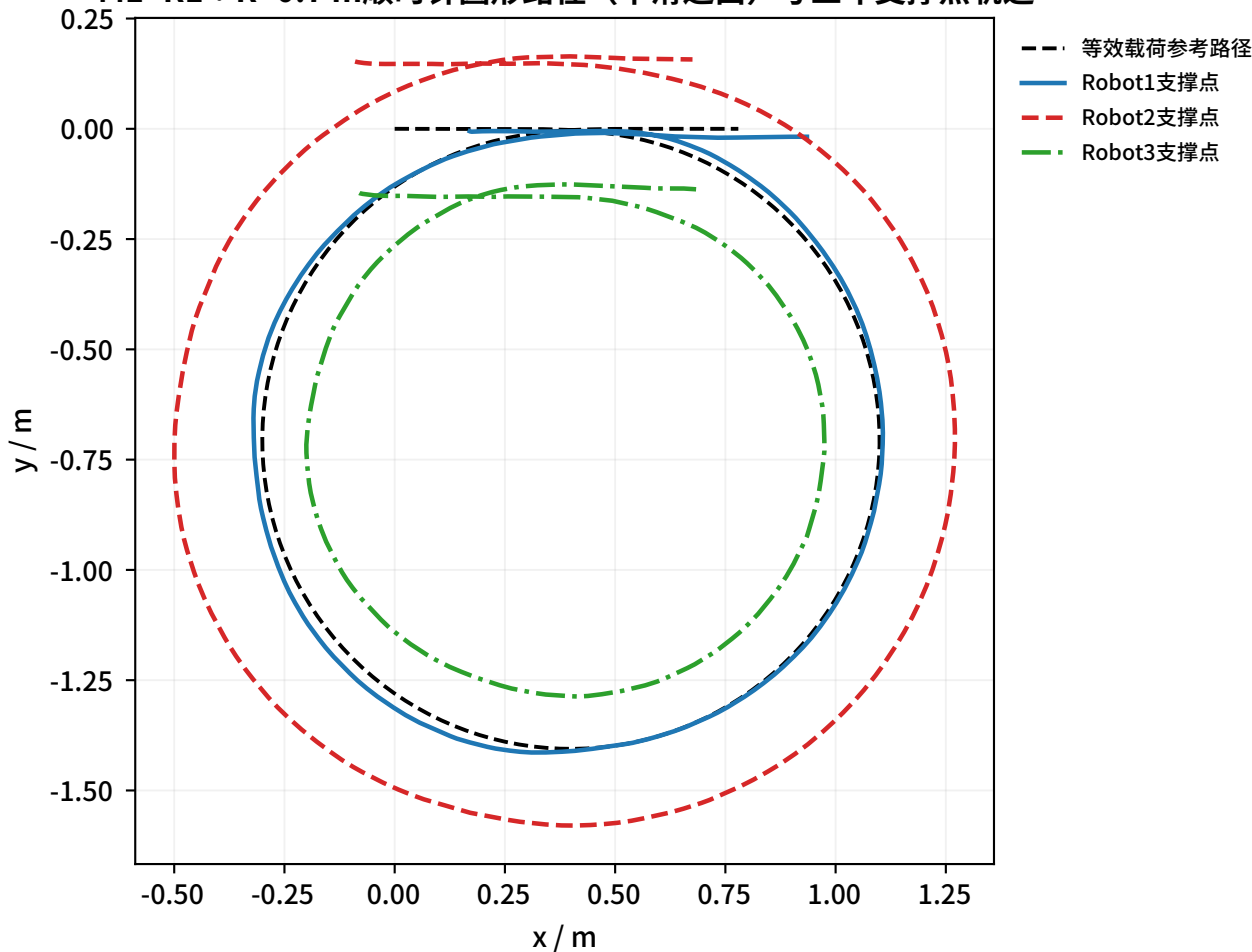
M1+R1 : R=0.7 m 顺时针圆形路径 (平滑进出) 与三车支撑点轨迹
