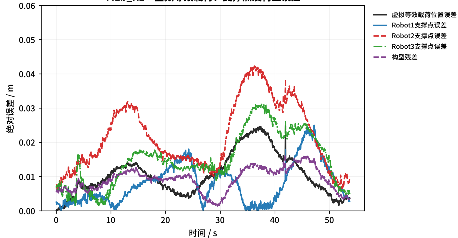
M1b_R1：虚拟等效载荷、支撑点及构型误差
