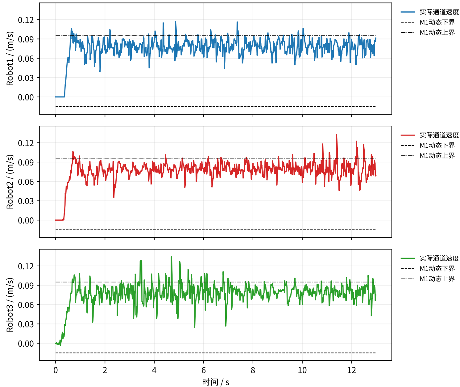
三车通道速度及M1动态上下界
