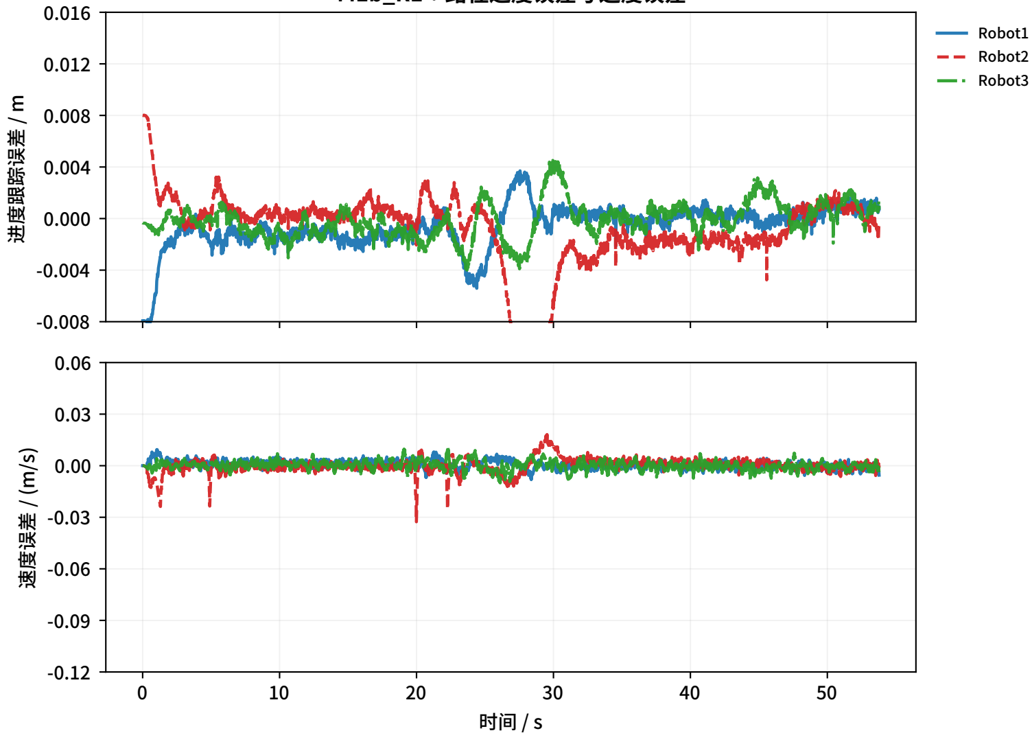
M1b_R1 : 路径进度误差与速度误差
