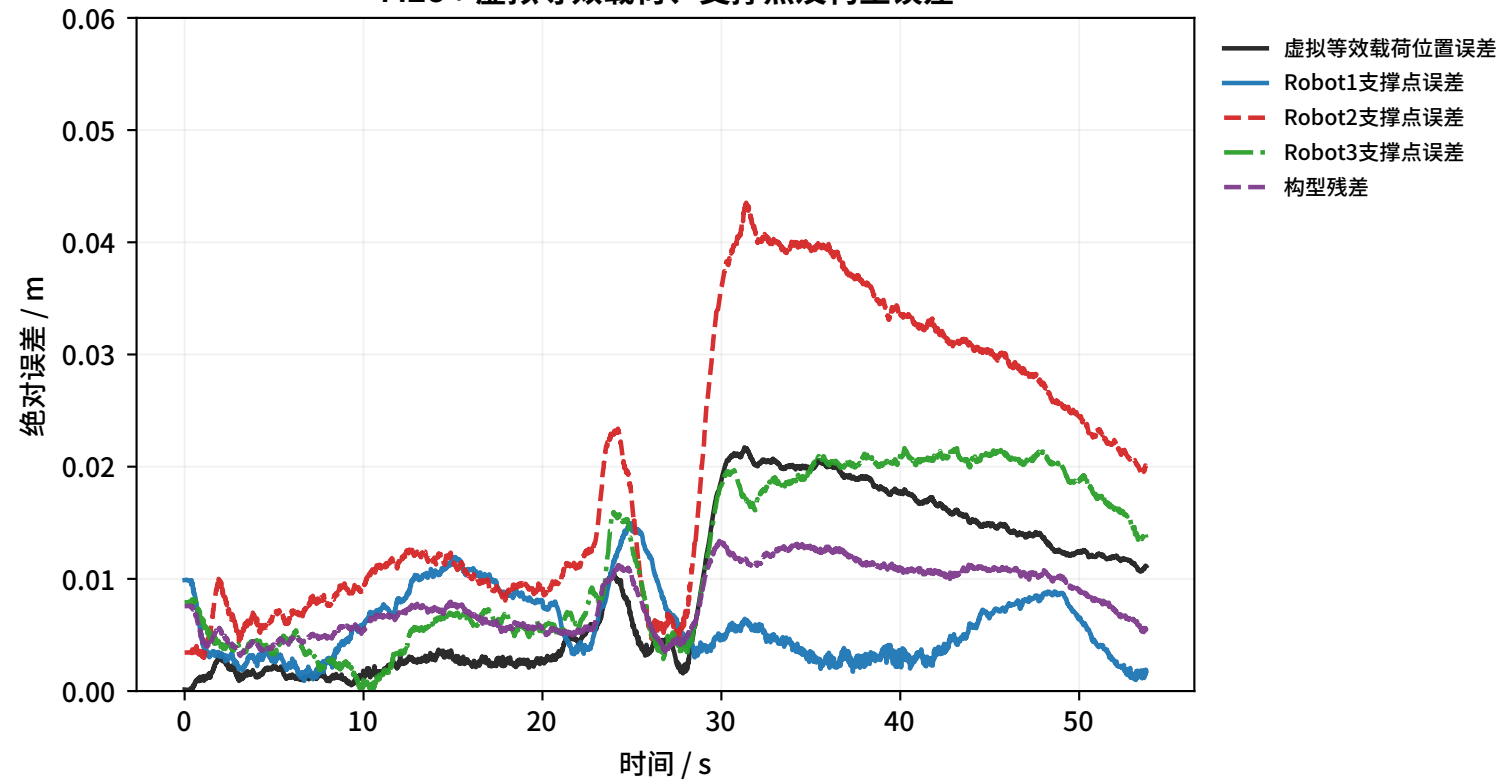
M2c：虚拟等效载荷、支撑点及构型误差
