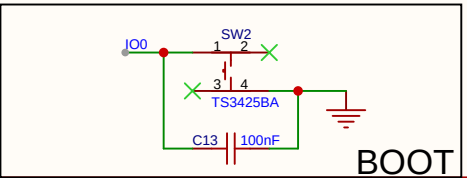
ESP32S3
