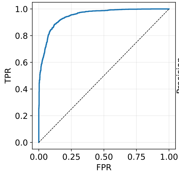
ROC (AUC=0.949)
