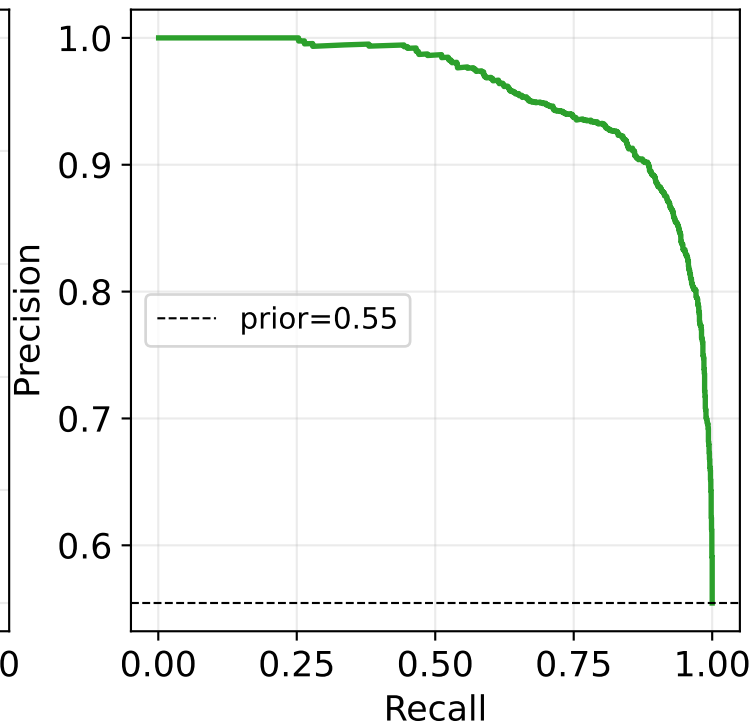
PR (AUC=0.958)
