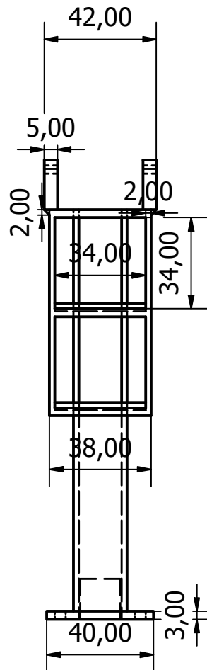
전면 ( 1 : 2 )
