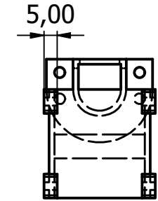
평면 ( 1 : 2 )
