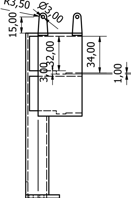
큰쪽 ( 1 : 2 )
