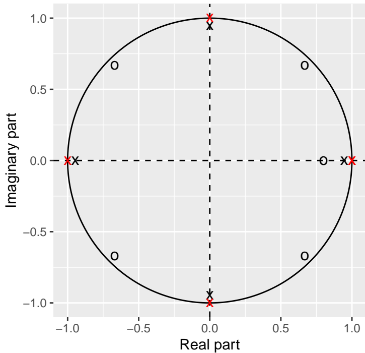
Poles (x – AR) and zeros (o – MA)
