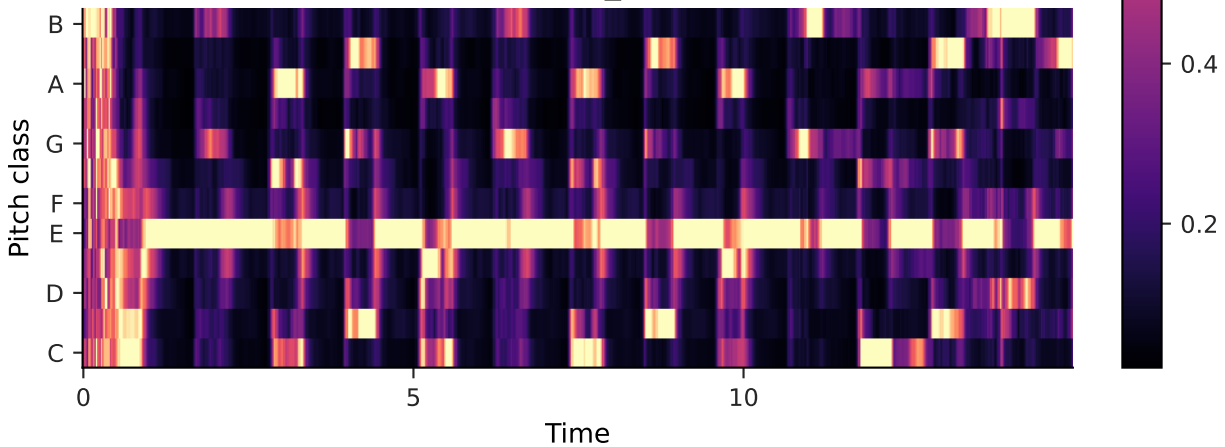
chroma_cqt
