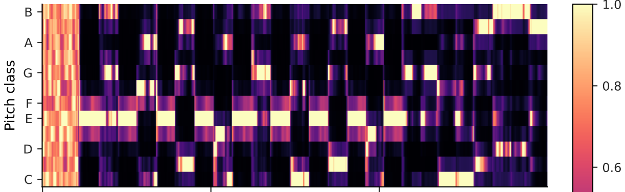
chroma_cqt
