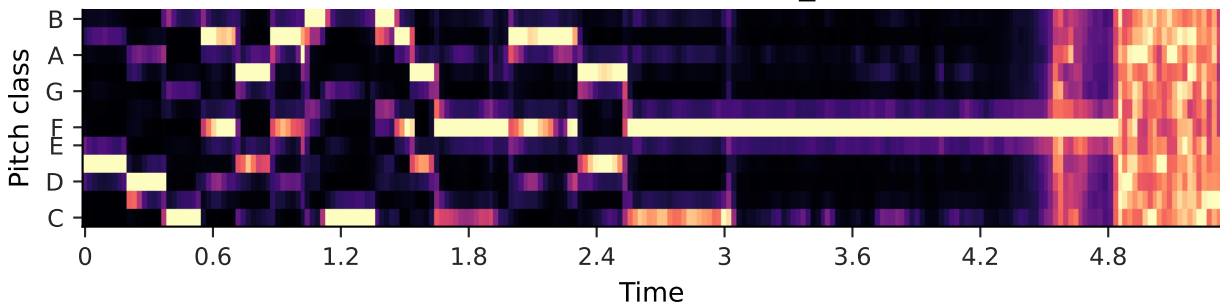
librosa.feature.chroma_stft
