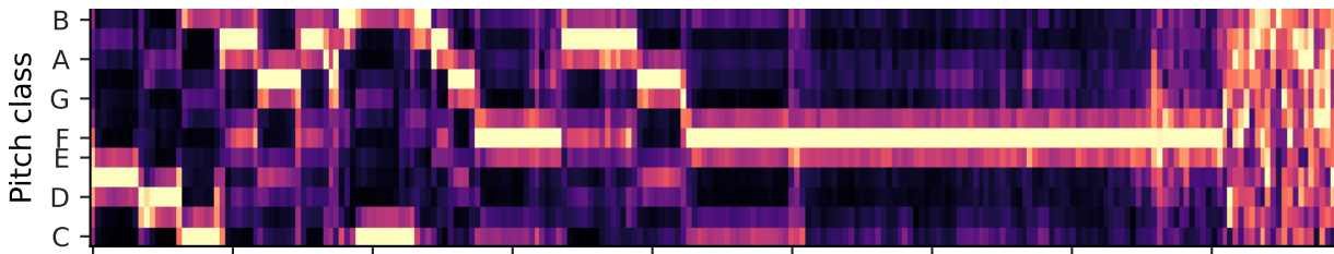
librosa.feature.chroma_stft
