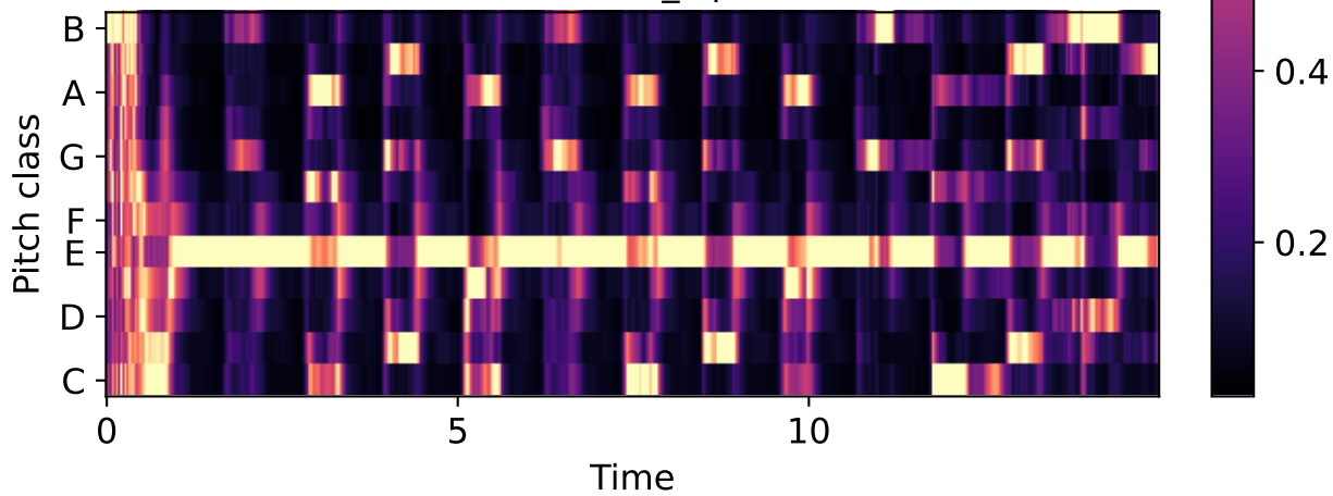
chroma_cqt
