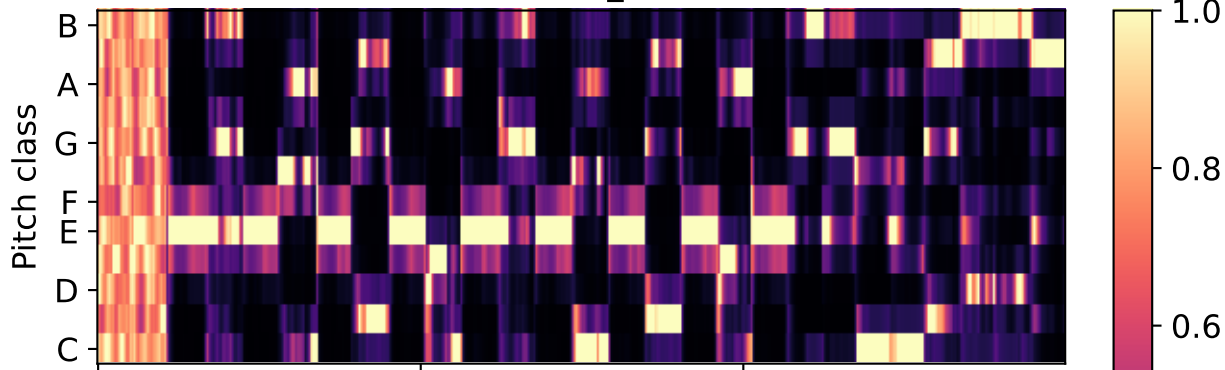
chroma_cqt
