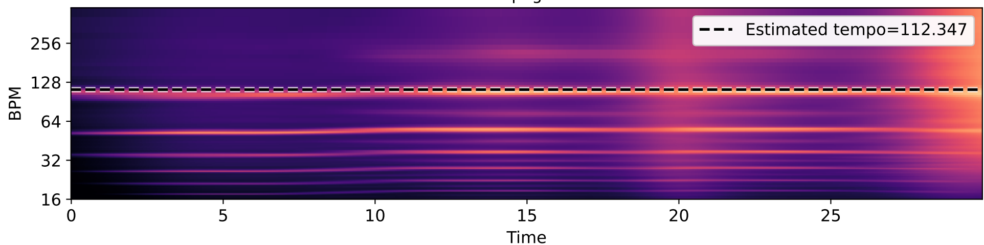
Tempogram
