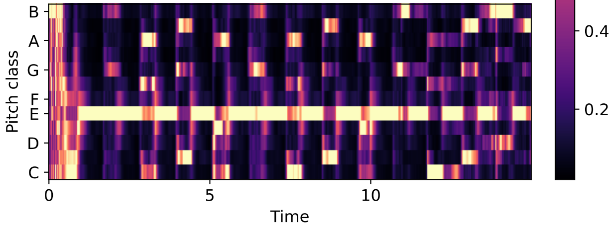
chroma_cqt
