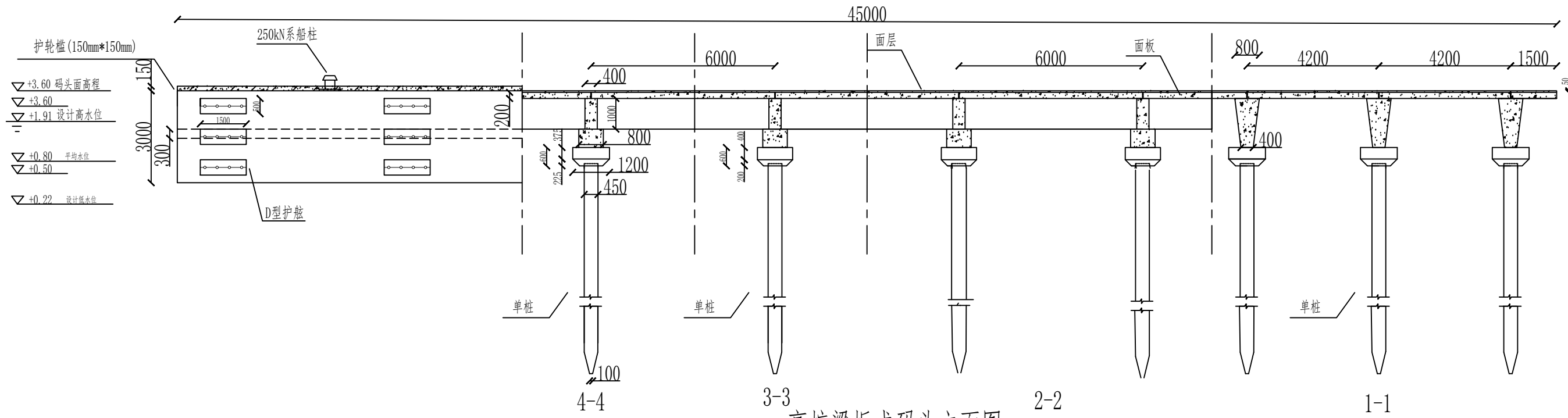
高桩梁板式码头立面图
