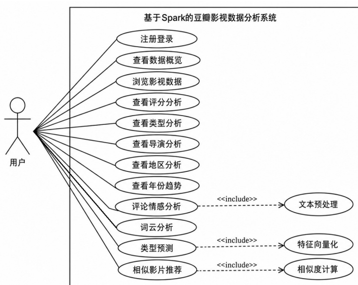
图 3-1 系统用户用例图
