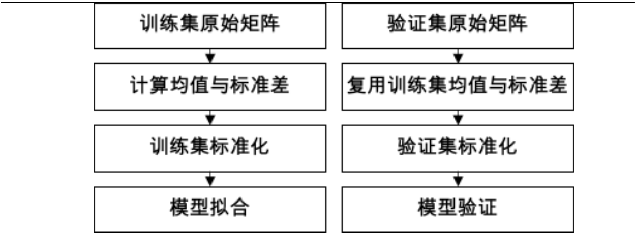
图 3.11 特征标准化流程图
