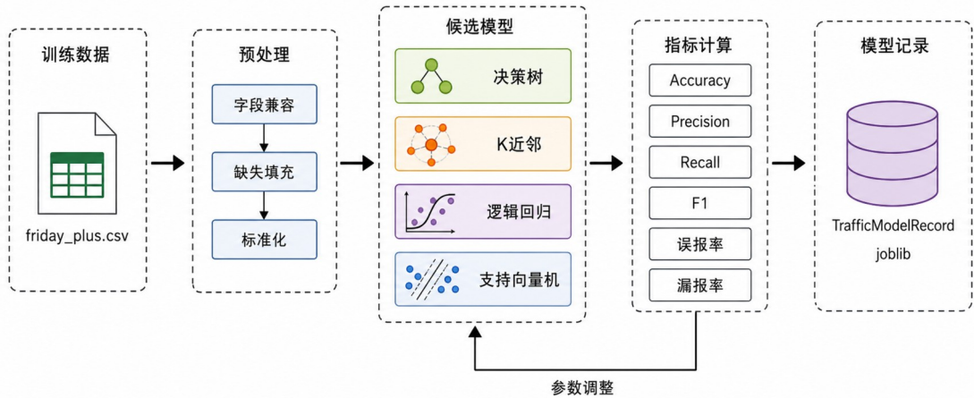
图 3.5 模型训练与评价流程图
