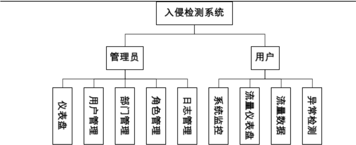
图 4.7 系统功能结构
