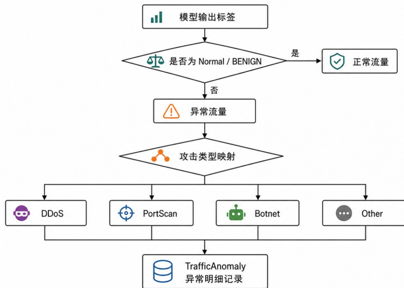
图 3.10 异常流量判定与落库流程
