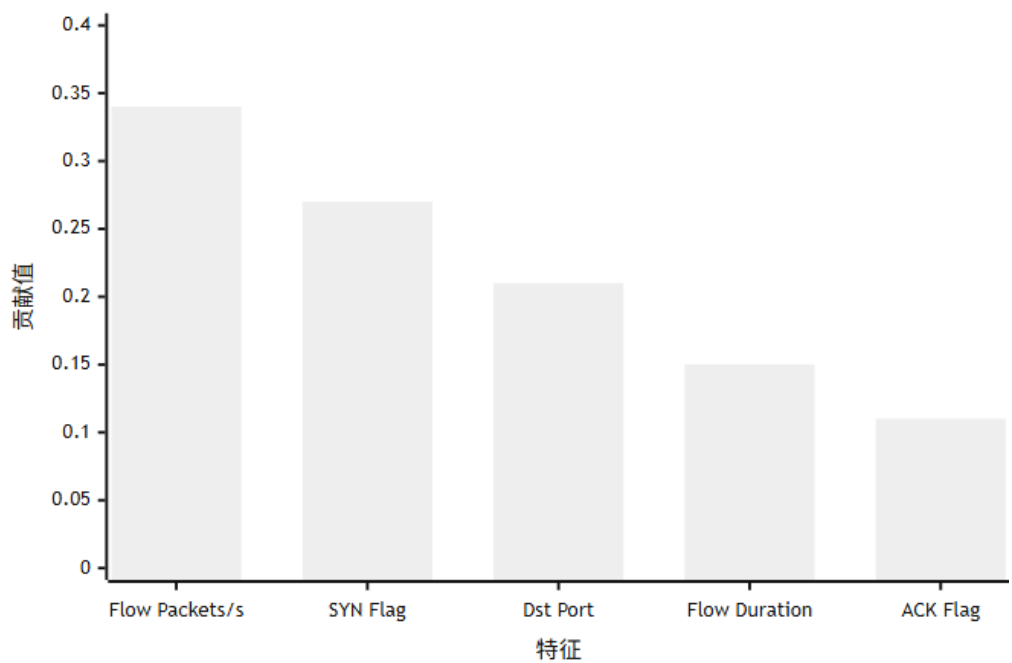
图 4.20 SHAP 式特征贡献排序图
