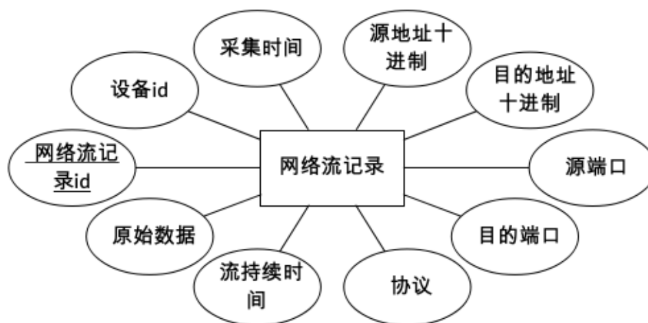
图 4.2 网络流记录实体属性图
