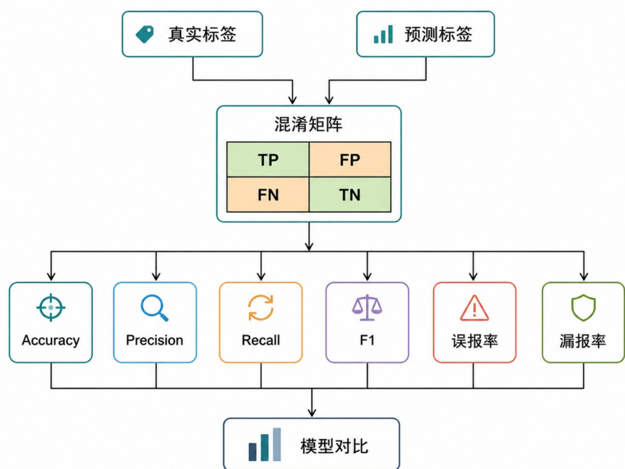
图 3.13 入侵检测模型评价指标结构
