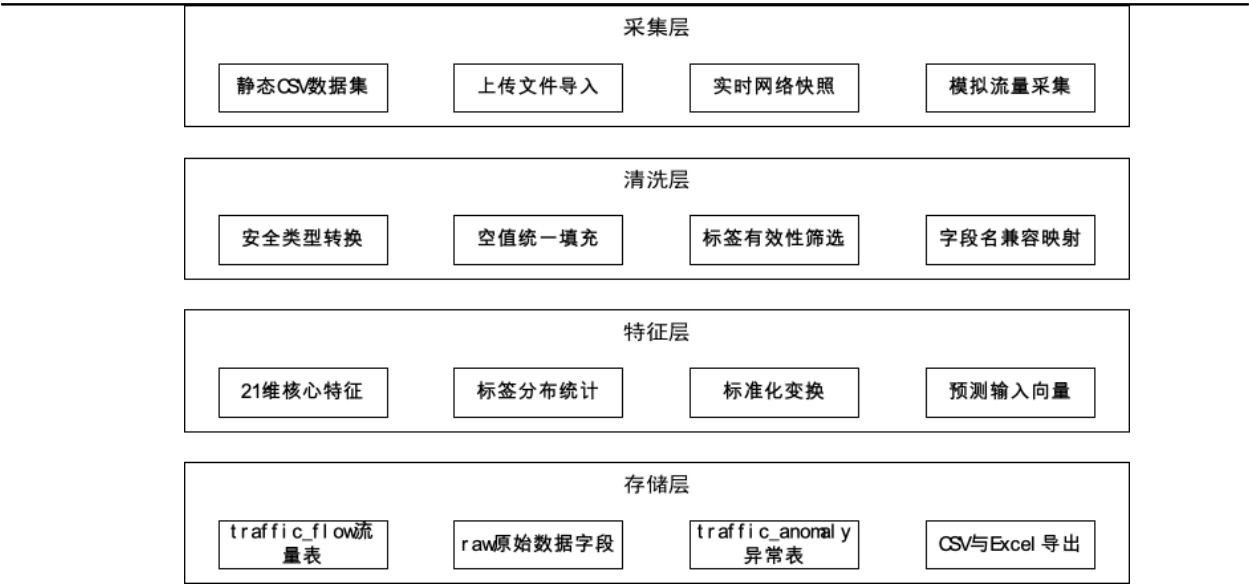
图 3.4 系统数据层架构图
