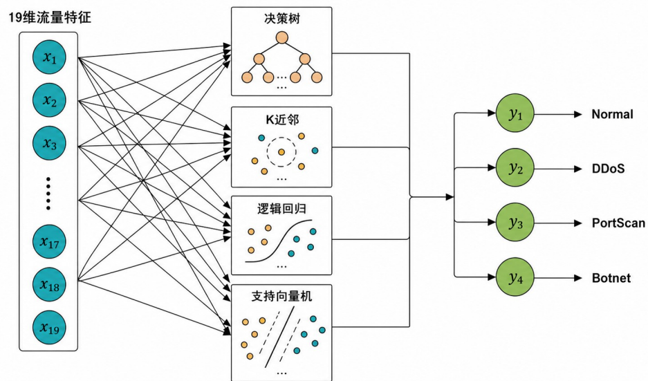
图 3.8 基于监督学习的多模型入侵检测结构
