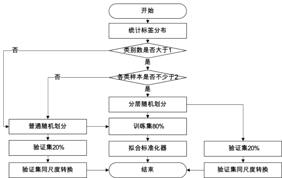
图 3.7 样本切分策略图
