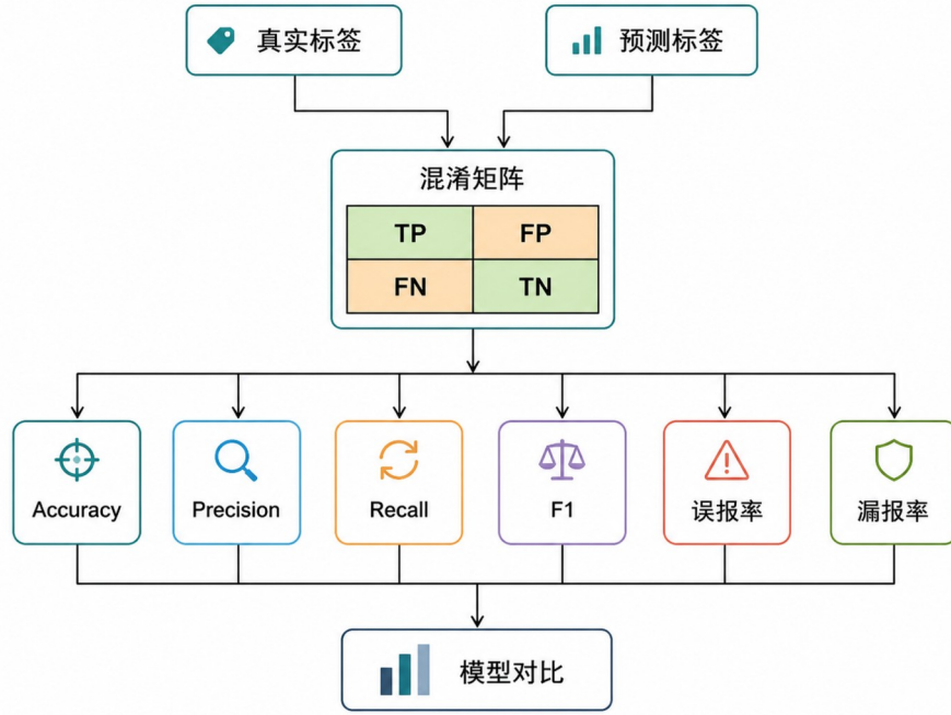
图 2.1 入侵检测模型评价指标结构
