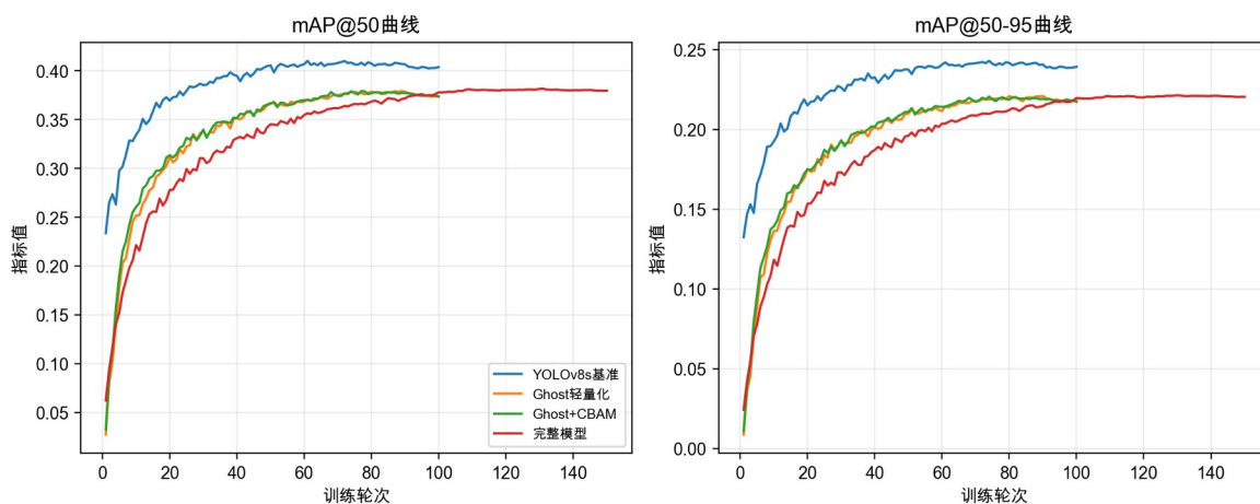
图 4.9 四类模型 mAP 曲线图
