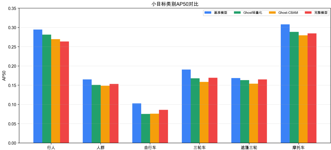
图 4.6 小目标类别 AP50 对比图
