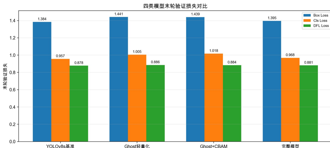
图 4.8 四类模型末轮验证损失对比图
