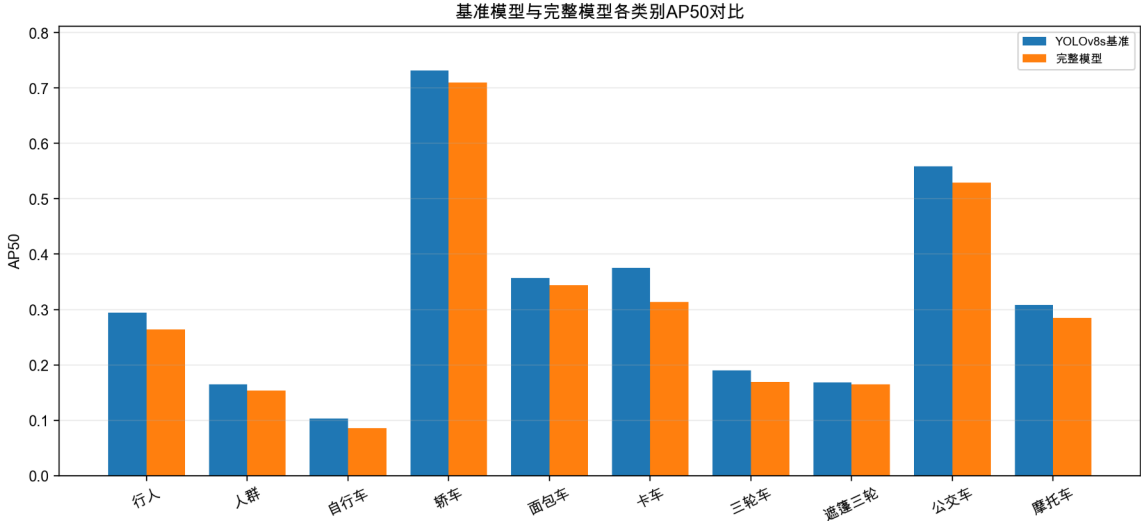
图 4.5 各类别 AP50 对比图
