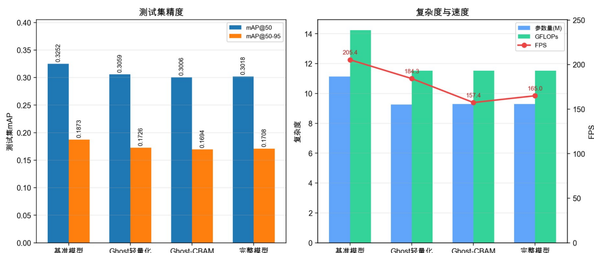
图 4.11 测试集综合评价图
