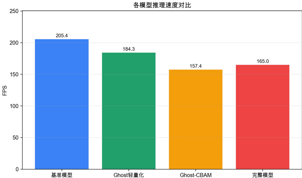
图 4.10 各模型推理速度对比图
