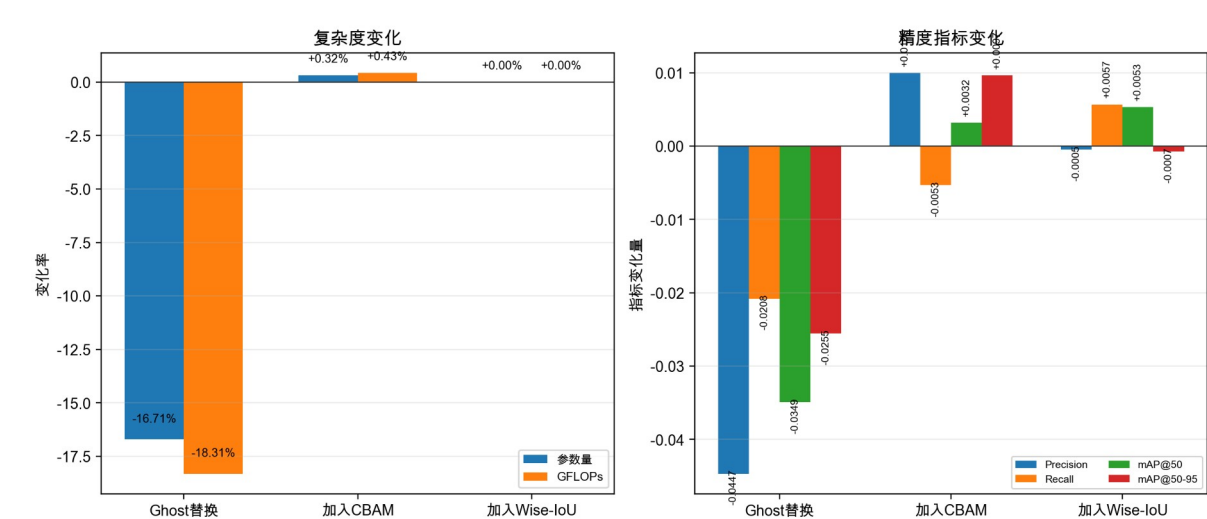
图 4.4 三类改进模块关键指标变化图
