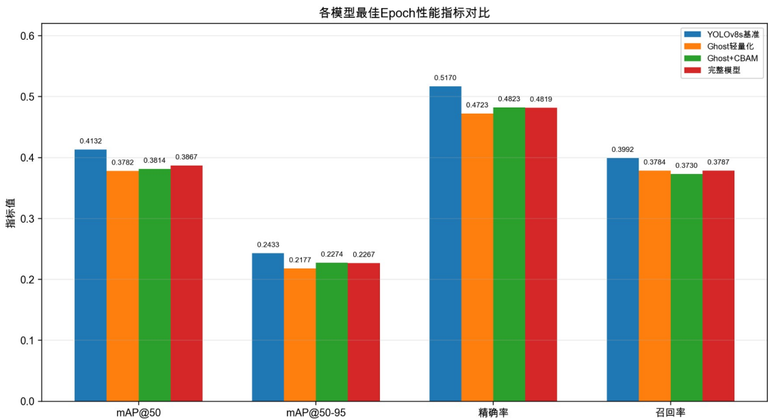
图 4.3 各模型最佳 Epoch 性能指标对比
