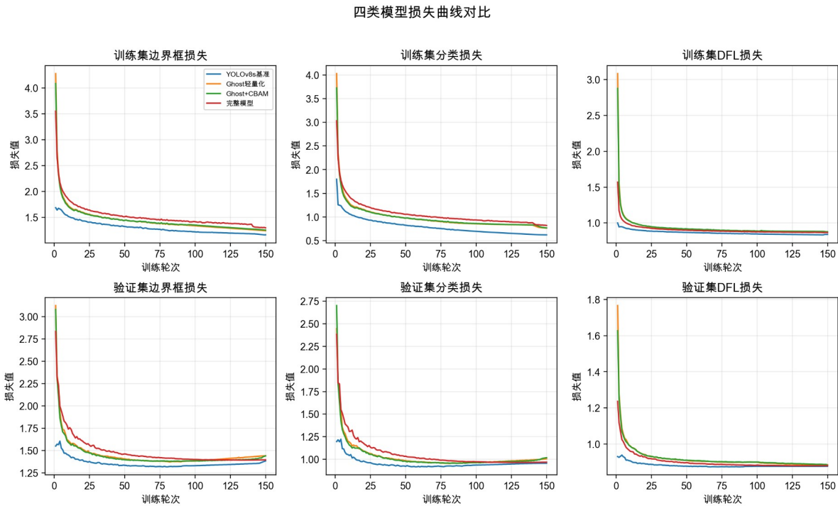
图 4.7 四类模型损失曲线图
