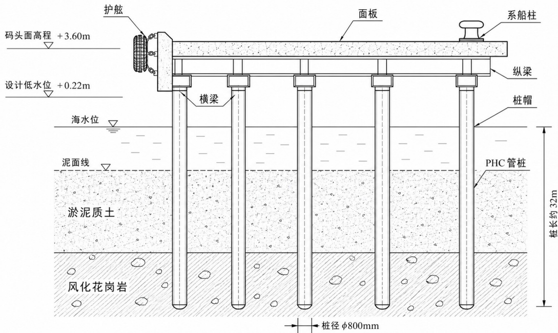
图 6-1 高桩梁板式码头结构断面图
