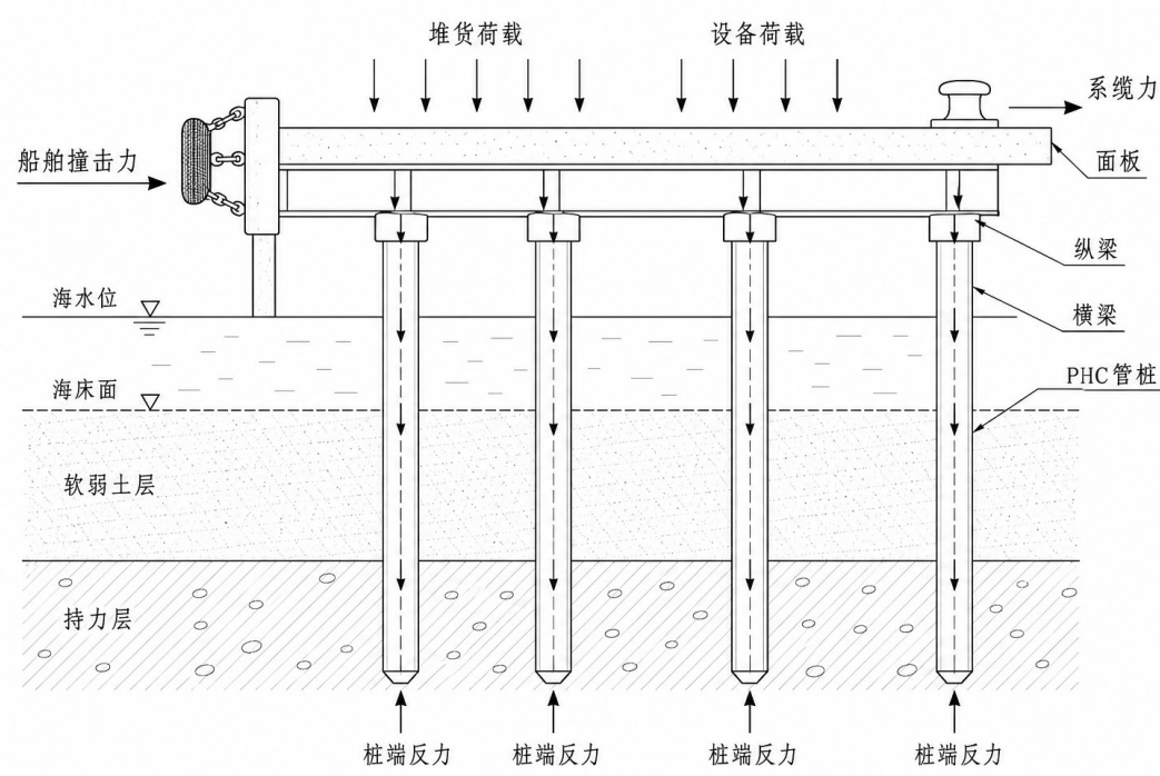
图 6-2 结构荷载与桩基传力图
