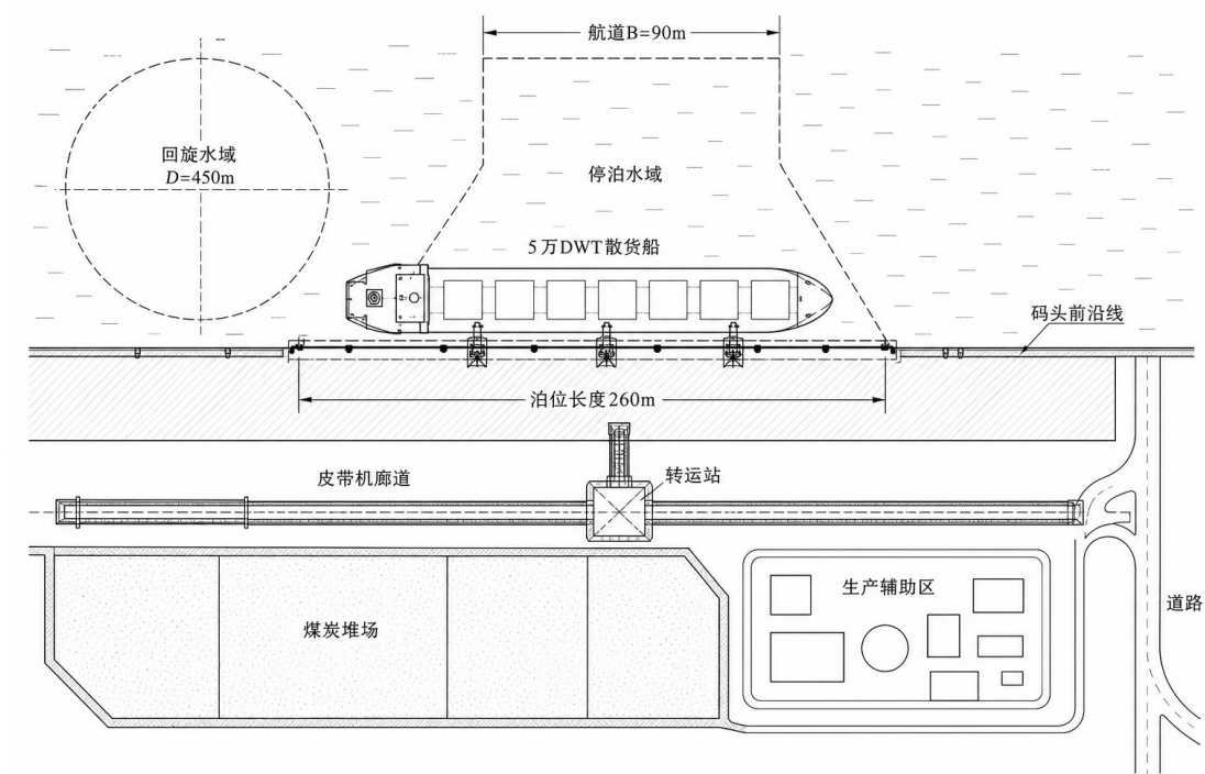
图 3-1 码头总平面布置图
