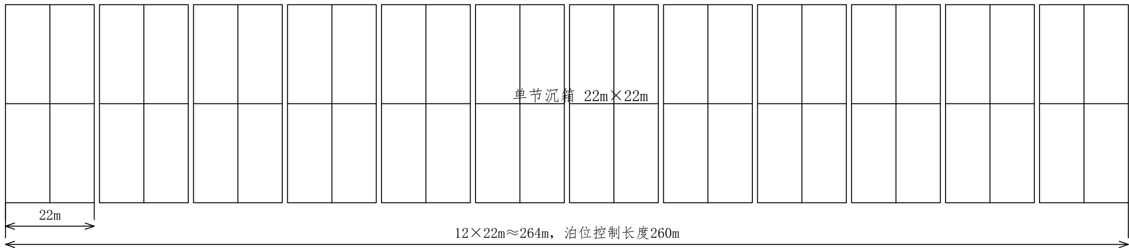
沉箱平面布置
