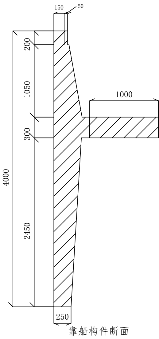
典型构件尺寸图
