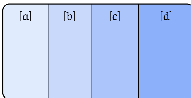
Figura 8: La relazione di equivalenza \sim determina la partizione \Omega = \{[a], [b], [c], [d]\} ; due elementi sono equivalenti se e solo se appartengono alla stessa classe.
