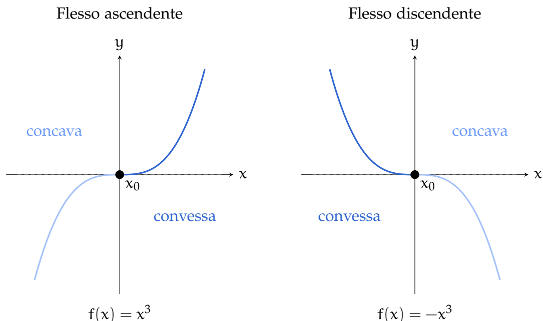
Figura 7.9: Il punto x_0 separa due intervalli con concavità opposta. In entrambi i casi il flesso è orizzontale e la tangente inflessionale ha equazione y = 0 .
