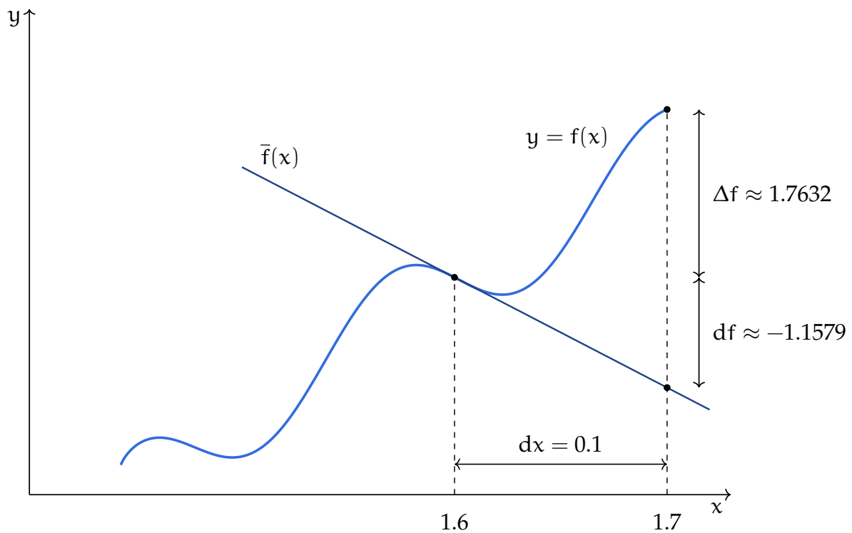
Figura 7.1: In figura è riportata l'approssimante lineare \bar{f}(x) per la funzione f(x) = 3x^2 + \sqrt{x^3 - 3} + \sin^2(25x) + 2 nel punto x_0 = 8/5 , sono riportati il differenziale df e la variazione \Delta f della funzione per dx = 0,1 .
