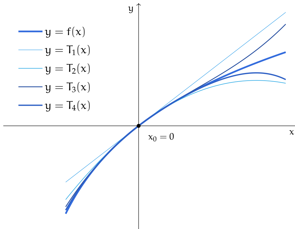
Figura 7.18: Polinomi di Taylor di y = \ln(x+1)
