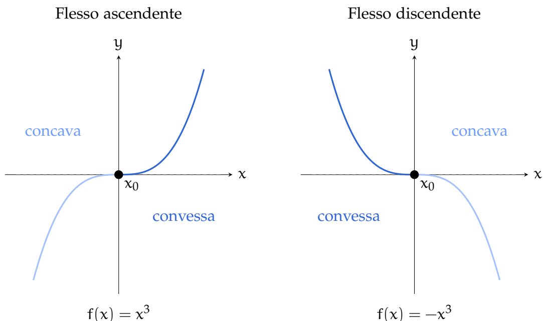
Figura 7.9: Il punto x_0 separa due intervalli con concavità opposta. In entrambi i casi il flesso è orizzontale e la tangente inflessionale ha equazione y = 0 .
