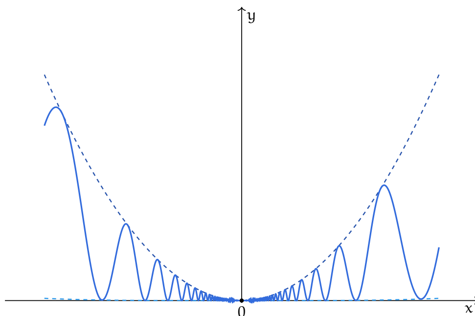
Figura 7.8: Il grafico della funzione f si trova compreso tra quello di f(x) = x^4 e quello di f(x) = x^2 per x \in [-1, 1] .
