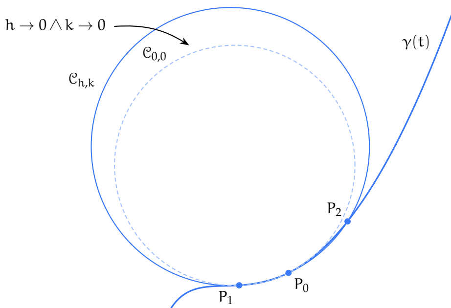
Figura 7.19: La circonferenza per tre punti C_{h,k} è definita dai parametri h e k introdotti per la costruzione di P_1 e P_2 . Al tendere di P_1 e P_2 a P_0 , C_{h,k} tende a C_{0,0} .
