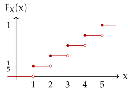
Funzione di ripartizione: ( n = 5 )
