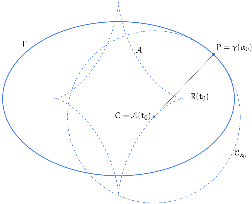
Figura 7.21: L'ellisse \Gamma , la sua astroide \mathcal{A} e il cerchio osculatore per \alpha_0 = 7\pi/36 . Il centro del cerchio osculatore giace sull'astroide, evoluta dell'ellisse.
