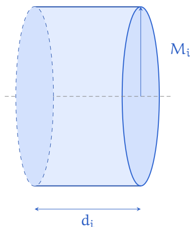
Figura 9.8: Il rettangolo i -esimo, ruotando attorno all'asse x , genera un cilindro di raggio M_i e altezza d_i . La misura del volume del pluri-cilindro è la somma delle misure dei singoli volumi.
