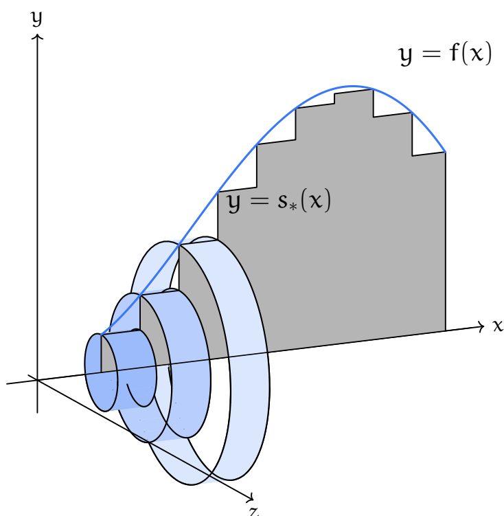
Figura 9.9: Pluri-cilindro generato dal pluri-rettangolo inscritto R_*
