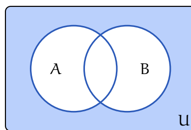
Figura 1: Formula di De Morgan per l'unione: (A \cup B)^c = A^c \cap B^c
