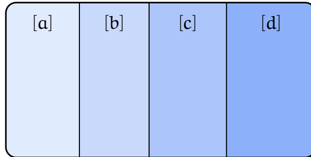
Figura 3: La relazione di equivalenza \sim determina la partizione \Omega = \{[a], [b], [c], [d]\} ; due elementi sono equivalenti se e solo se appartengono alla stessa classe.
