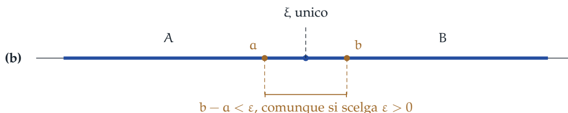
Figura 2.1: Classi separate e classi contigue. Nel primo caso gli elementi separatori riempiono un intervallo; nel secondo si riducono a uno solo.
