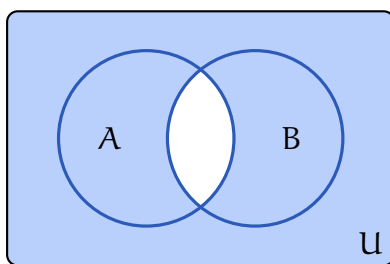
Figura 2: Formula di De Morgan per l'intersezione: (A \cap B)^c = A^c \cup B^c
