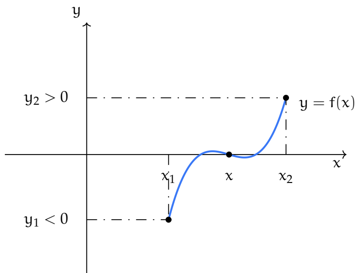
Figura 5.2: Teorema degli zeri
