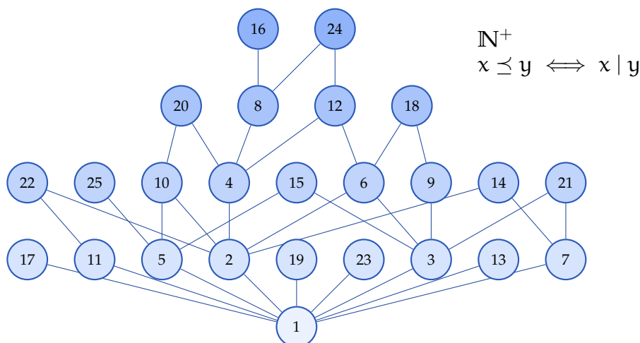
Figura 8: Frammento del diagramma di Hasse di (\mathbb{N}^+, |) . Un numero posto più in alto è divisibile per quelli collegati sotto; un arco di copertura da a a b indica che b/a è primo.
