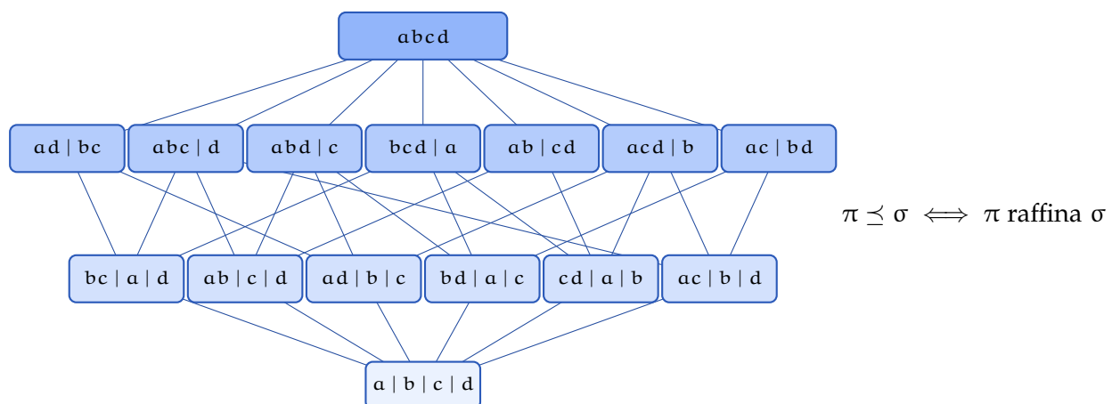
Figura 7: Diagramma di Hasse delle 15 partizioni di \{a, b, c, d\} ordinate per raffinamento. Le barre separano i blocchi: una partizione con meno blocchi è posta più in alto ed è maggiore.
