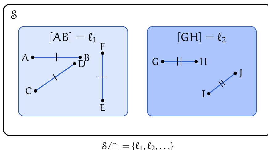
Figura 4: Due segmenti sono equivalenti quando sono congruenti. La lunghezza di un segmento AB è la sua classe di equivalenza [AB] rispetto a \cong .
