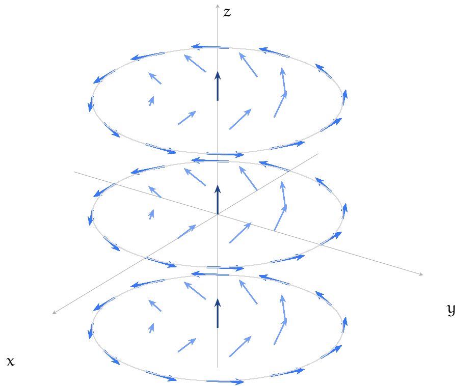
Figura G.1: In figura alcuni vettori del campo F(x, y, z) = (-y, x, \frac{3}{4}(1 - x^2 - y^2)) .
