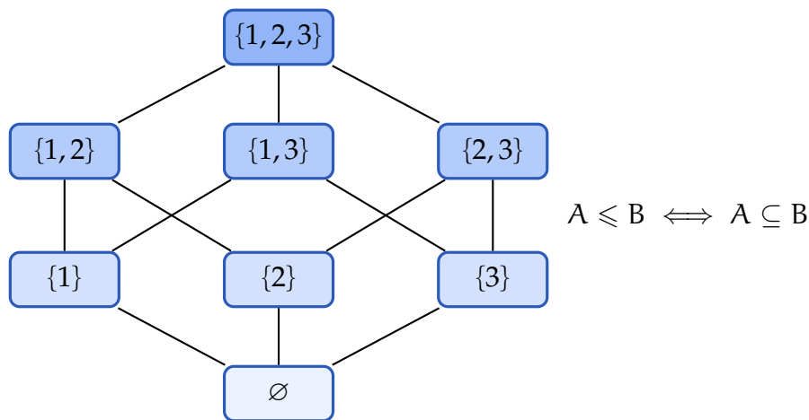
Figura 6: Diagramma di Hasse (\mathcal{P}(\{1,2,3\}), \subseteq) . Un insieme posto più in alto contiene quello collegato immediatamente sotto.
