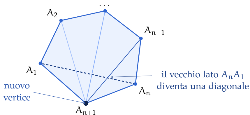
Figura 9: Nel passaggio da n a n + 1 vertici compaiono n - 2 diagonali uscenti dal nuovo vertice e una diagonale ottenuta dal vecchio lato A_n A_1 : in totale si aggiungono n - 1 diagonali.
