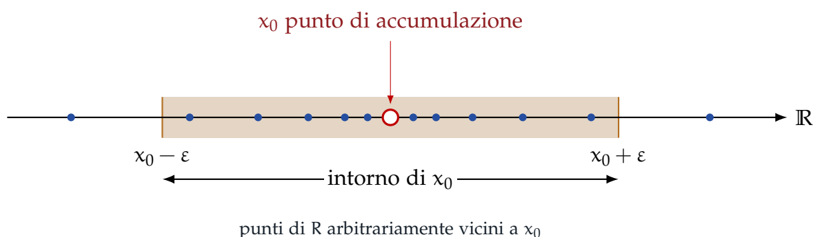
Figura 2.4: x_0 = 0 è l'unico punto di accumulazione per l'insieme R .
