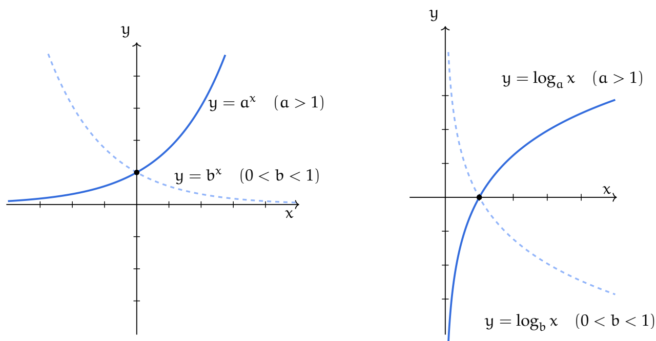
Figura 1.11: Grafici di funzioni esponenziali e logaritmiche
