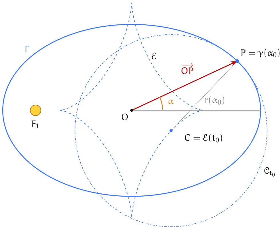
Figura 7.22: Il Sole si trova in F_1 ; quando \alpha = \pi il pianeta è al perielio, C è il centro istantaneo di rotazione, C la circonferenza istantanea lungo cui avviene la rotazione.
