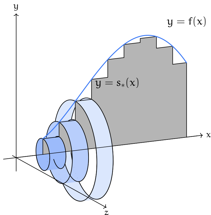
Figura 9.9: Pluri-cilindro generato dal pluri-rettangolo inscritto R_*
