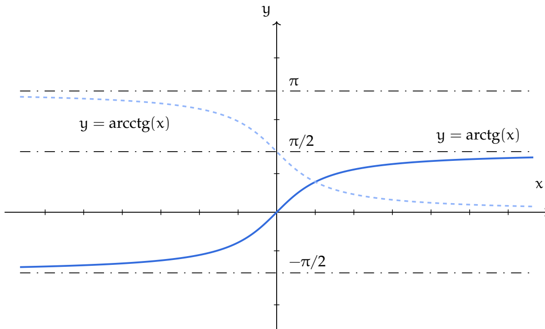
Figura 1.15: Grafici di arcotangente e arcocotangente
