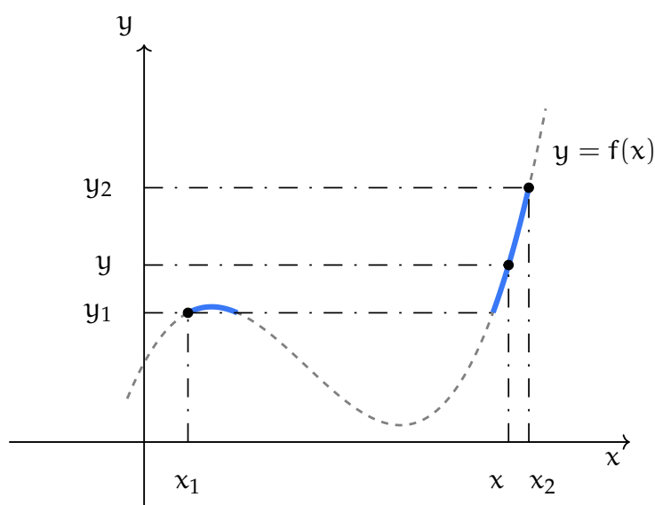
Figura 5.1: Teorema dei valori intermedi
