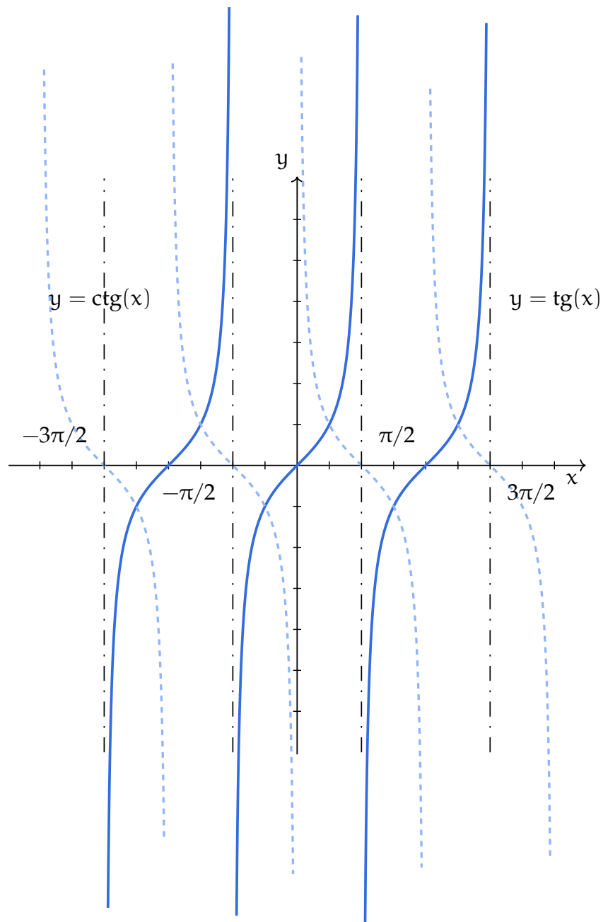
Figura 1.14: Grafici di tangente e cotangente
