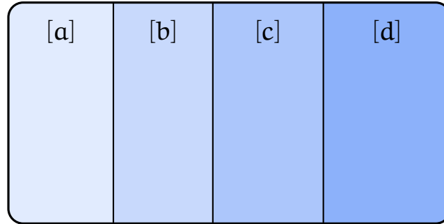
Figura 3: La relazione di equivalenza \sim determina la partizione \mathfrak{Q} = \{[a], [b], [c], [d]\} ; due elementi sono equivalenti se e solo se appartengono alla stessa classe.
