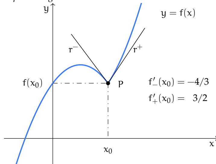
Figura 6.1: Punto angoloso per y = f(x)
