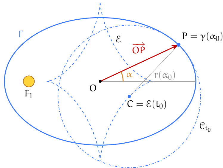
Figura 7.22: Il Sole si trova in F_1 ; quando \alpha = \pi il pianeta è al perielio, C è il centro istantaneo di rotazione, \mathcal{C} la circonferenza istantanea lungo cui avviene la rotazione.
