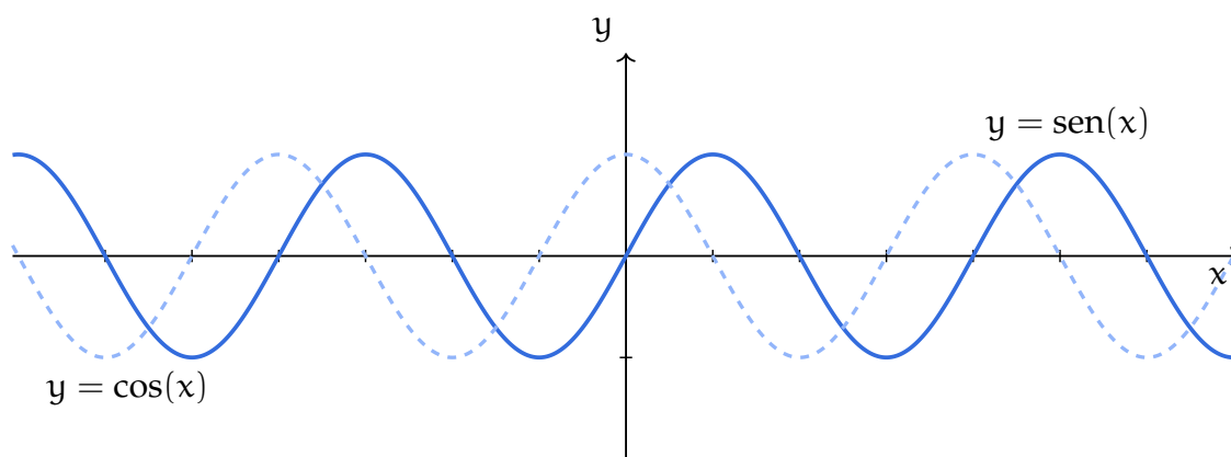
Figura 1.12: Grafici di seno e coseno
