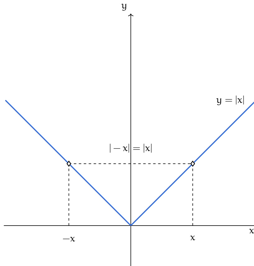
Figura 1.16: Grafico della funzione valore assoluto
