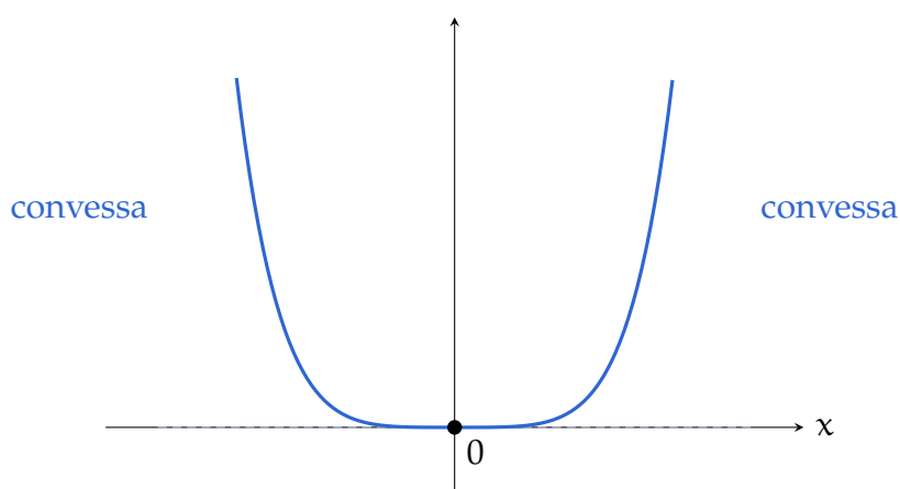
Figura 7.12: L'annullamento di h'' nell'origine non produce un flesso, perché la concavità non cambia: h''(0) = 0 , ma x_0 = 0 non è punto di flesso per h .
