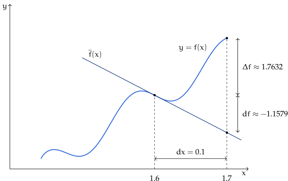
Figura 7.1: In figura è riportata l'approssimante lineare \bar{f}(x) per la funzione f(x) = 3x^2 + \sqrt{x^3 - 3} + \sin^2(25x) + 2 per il punto x_0 = 8/5 , sono riportati il differenziale df e la variazione \Delta f della funzione per dx = 0.1
