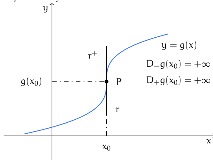
Figura 6.2: Punto di inflessione per y = g(x)
