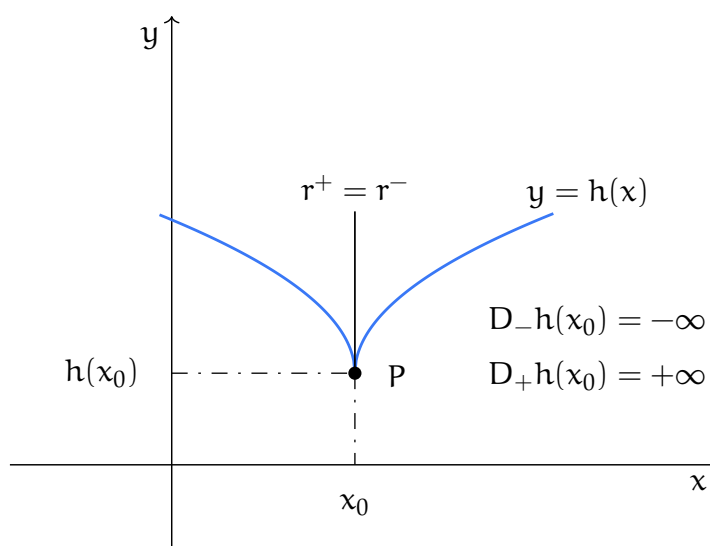
Figura 6.3: Punto cuspidale per y = h(x)
