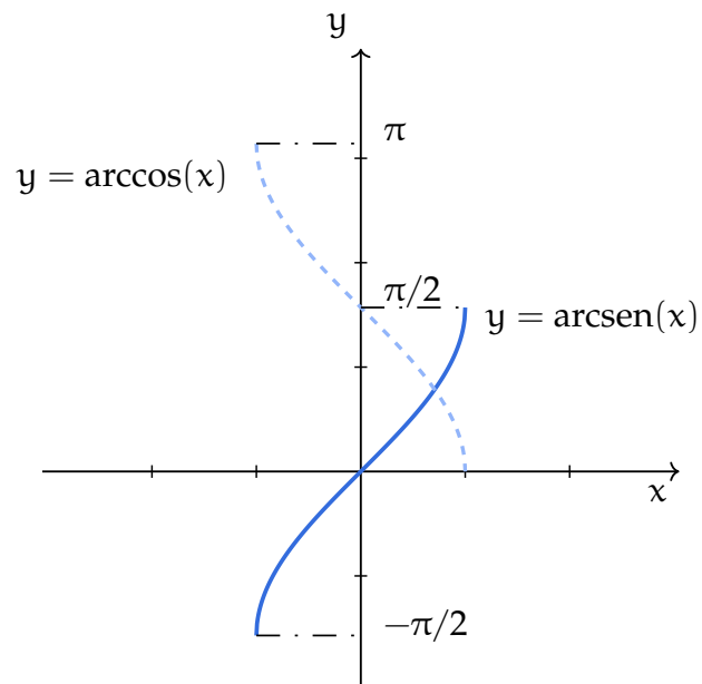
Figura 1.13: Grafici di arcoseno e arcocoseno
