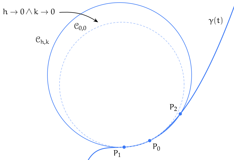
Figura 7.19: Il cerchio per tre punti \mathcal{C}_{h,k} è definito dai parametri h e k introdotti per la costruzione di P_1 e P_2 . Al tendere di P_1 e P_2 a P_0 , \mathcal{C}_{h,k} tende a \mathcal{C}_{0,0} .
