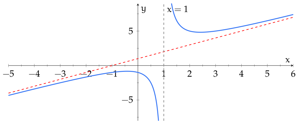
Figura 7.14: Grafico della funzione con gli asintoti verticale e obliquo
