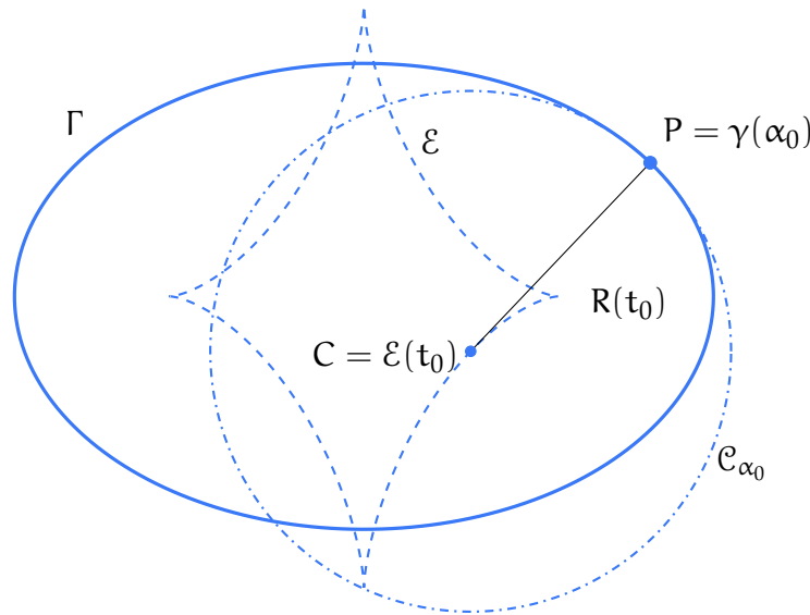
Figura 7.21: L'ellisse \Gamma , la sua astroide \varepsilon , e il cerchio osculatore per \alpha_0 = 7\pi/36 . Il centro del cerchio osculatore giace sull'astroide, evoluta dell'ellisse.
