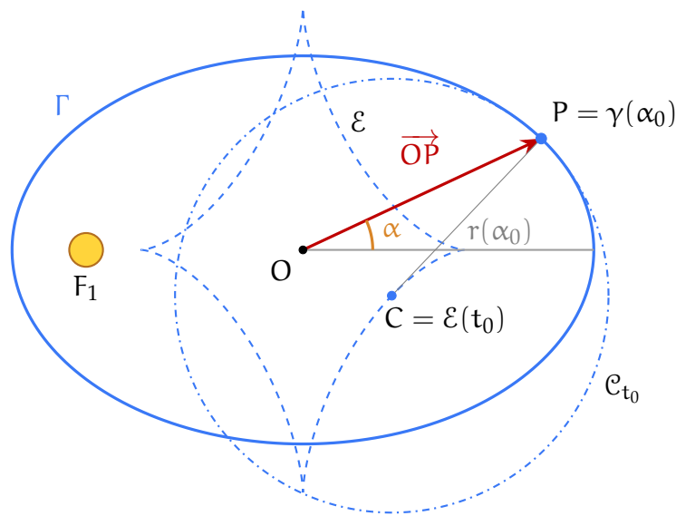
Figura 7.22: Il Sole si trova in F_1 ; quando \alpha = \pi il pianeta è al perielio, C è il centro istantaneo di rotazione, \mathcal{C} la circonferenza istantanea lungo cui avviene la rotazione.
