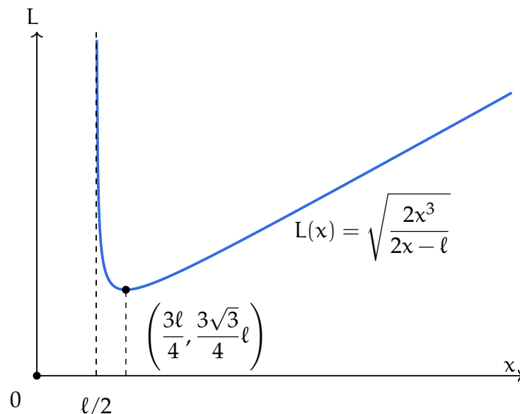
Figura 7.3: La funzione L(x) presenta un minimo in x = 3\ell/4 , per tale valore la piega ha quindi lunghezza minima
