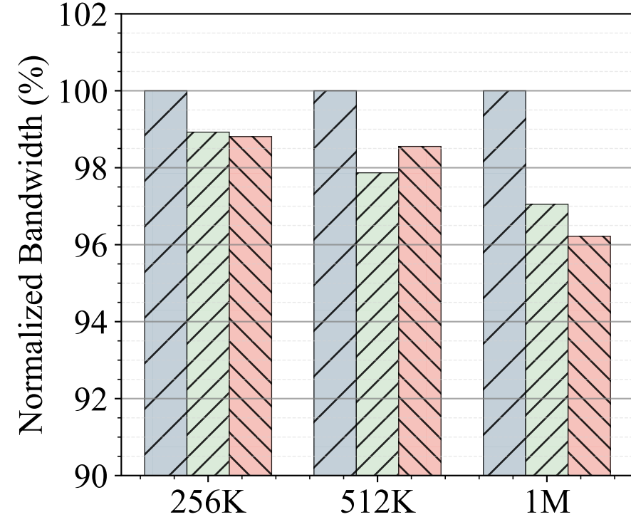
(d) Sequential Write Bandwidth
