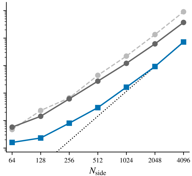
spin 2
