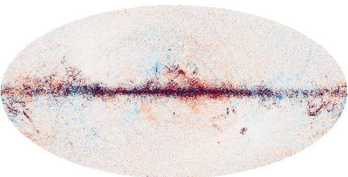
NPIPE A 857 GHz
