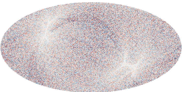
NPIPE A 143 GHz
