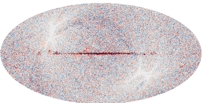
NPIPE A 217 GHz
