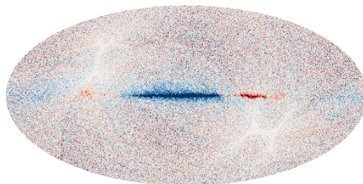
FFP10 HM1 857 GHz
