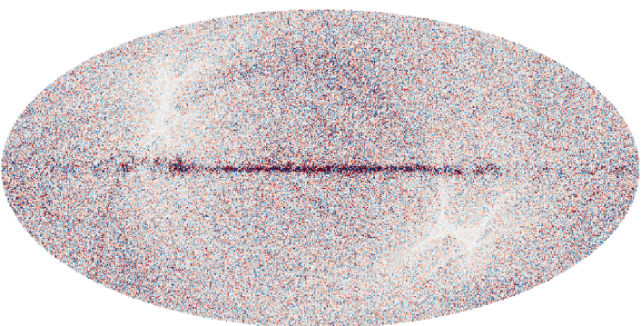
NPIPE A 353 GHz
