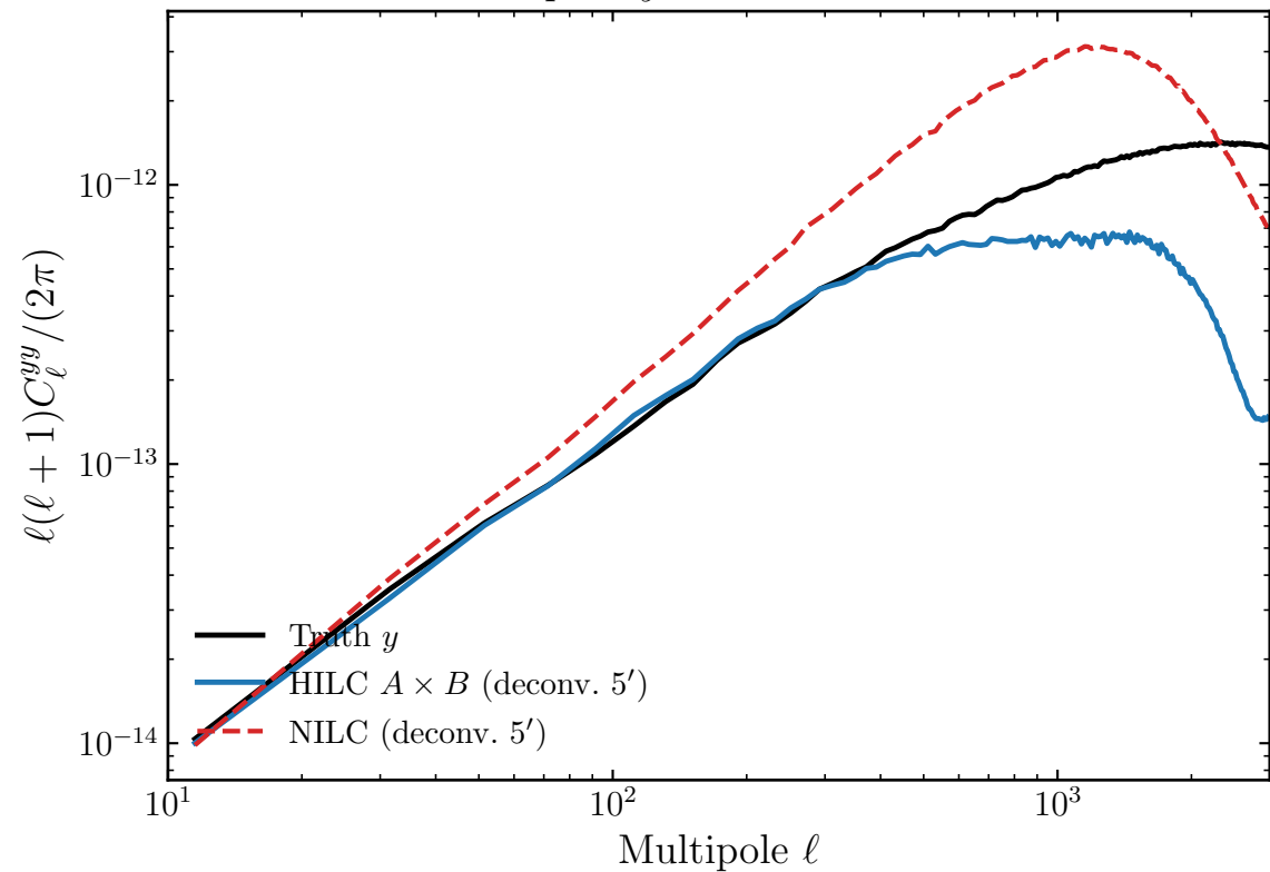
ILC Compton- y vs FLAMINGO truth
