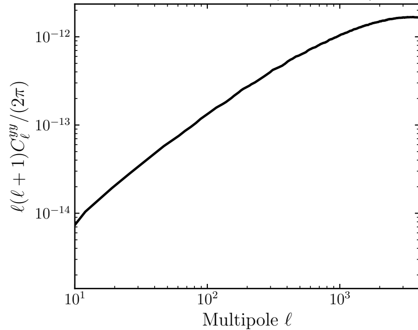
tSZ auto-spectrum (Compton y )
