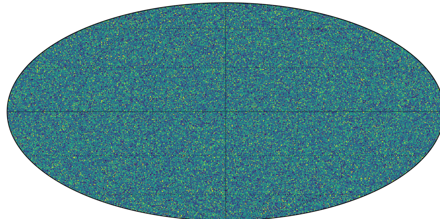
CIB \Delta T — 857 GHz
