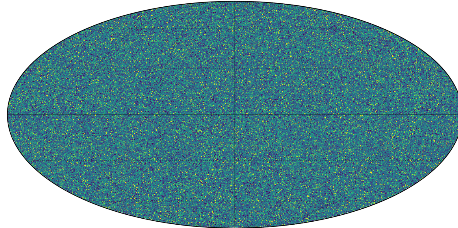
CIB \Delta T — 217 GHz
