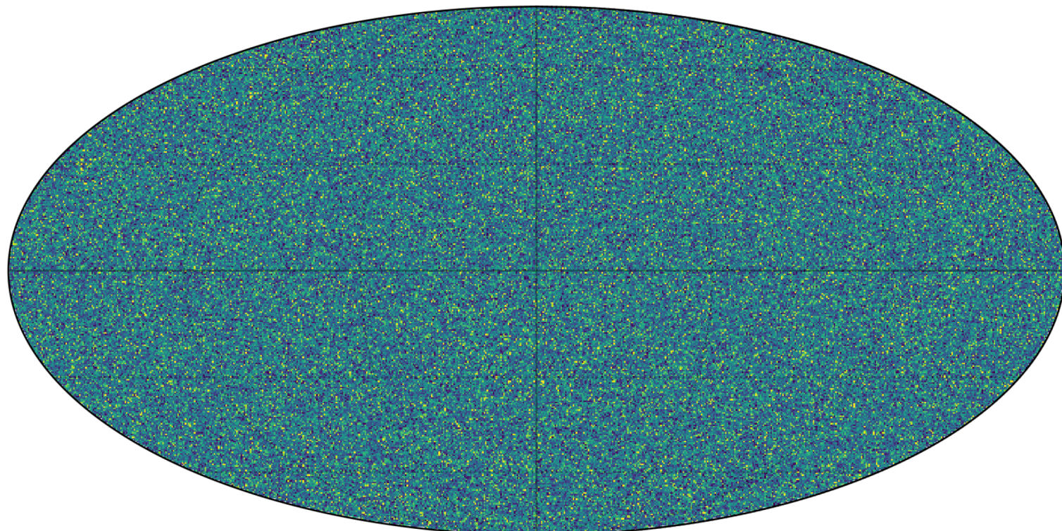
CIB \Delta T — 353 GHz
