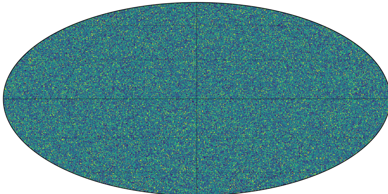
CIB \Delta T — 545 GHz
