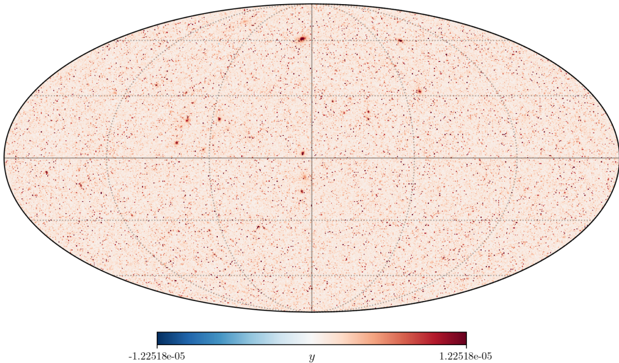
Compton y (lensed tSZ)
