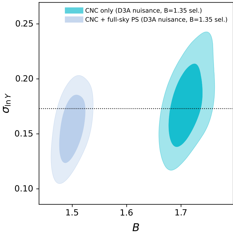
D3A nuisance, B=1.35 sel.: B vs sigma_lnY
