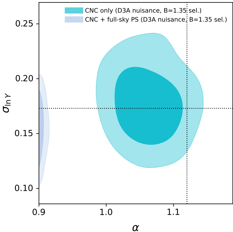
D3A nuisance, B=1.35 sel.: alpha_SZ vs sigma_lnY
