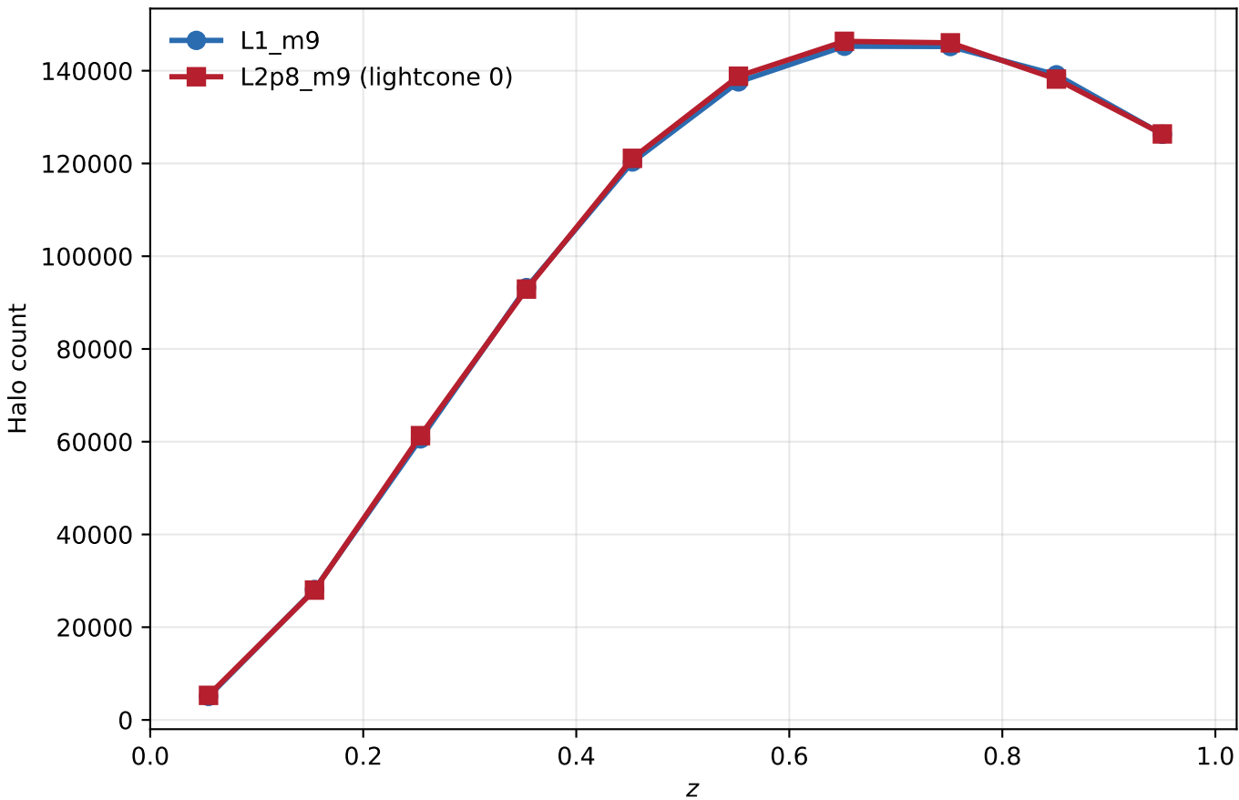
z histogram ( M_{500c} > 5 \times 10^{13} M_{\odot} )
